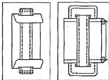
а) б) Рис. 4.23. Настрачивание шлевки (а) и отделочной накладки (б)
