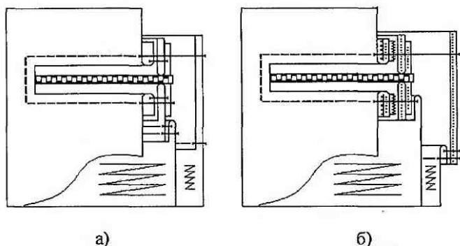
Рис. 4.37. Обработка прорезного кармана в рамку с тесьмой молнией ниточным (а) и клеевым (б) способом
