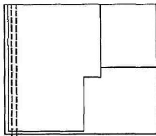
Рис. 4.13. Обработка верхней части шлицы обтачкой
