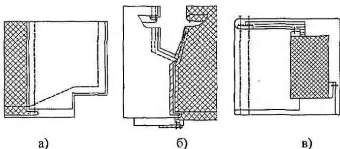
Рис. 4.86. Обработка низа изделия с притачной подкладкой: а — обработка нижнего угла борта; б — соединение подкладки с припусками на обработку шлицы; в — притачивание подкладки по низу
