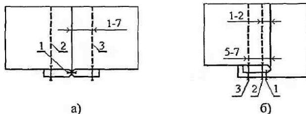
Рис. 4.6. Обработка рельефов ниточным способом в изделиях из толстых (а) и тонких кож (б)
