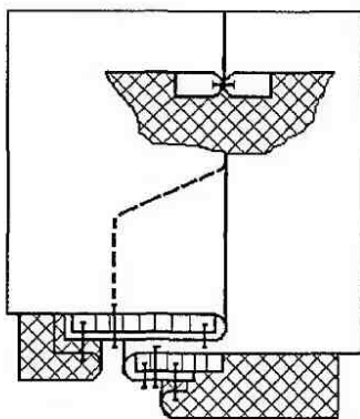
Рис. 4.9. Обработка шлицы
