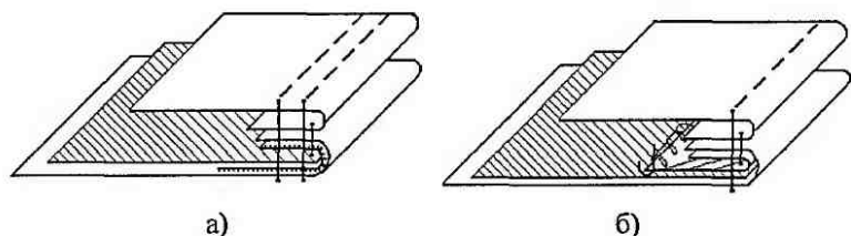
Рис. 4.48. Обработка края борта в изделиях из тонкой кожи и замши с лейкопластырем (а) и кромкой (б)
