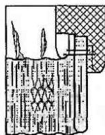
Рис. 4.80. Обработка низа рукавов трикотажными манжетами
