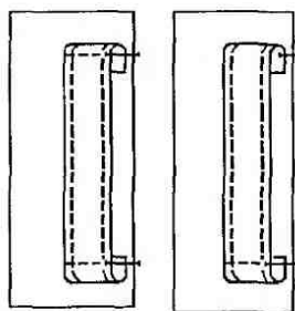
а) б) Рис. 4.22. Варианты соединения шлевки с изделием:
