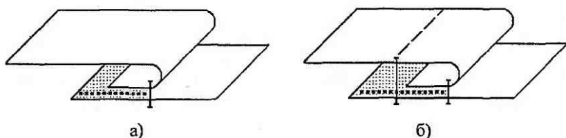
Рис. 3.2. Стачной шов взаютуюжку (а) и настрочной шов с закрытым срезом (б)
