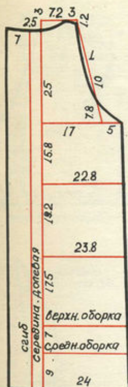
Спинка-2 дет.
