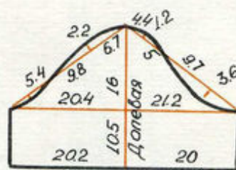
Рукав-2дет.
