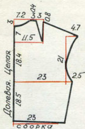
Спинка жакета-идет.
