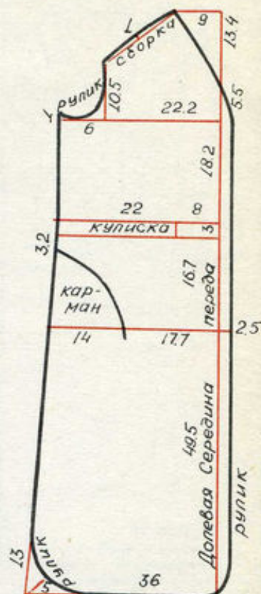
Полочка-2дет.
