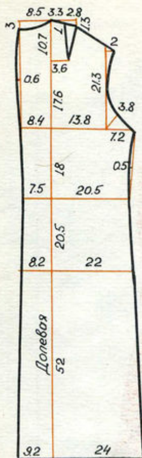
Спинка-2дет.
