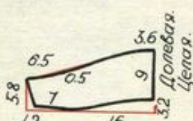
Воротник-1дет.
