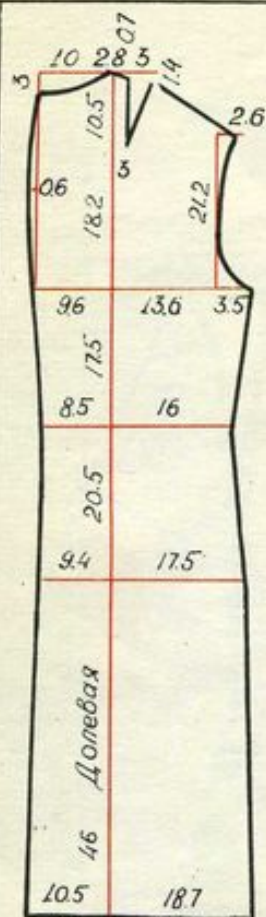
Спинка-2дет.
