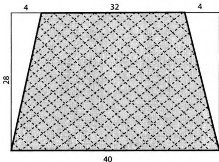
задняя часть 1 дет.
