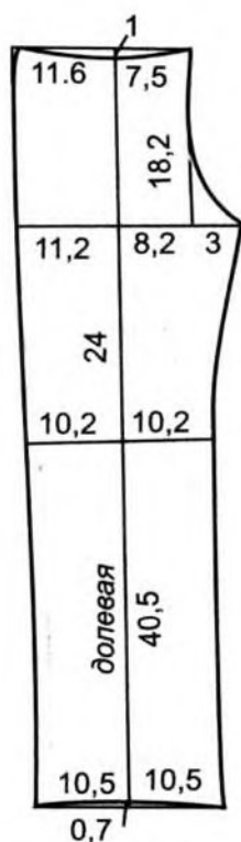
передняя половинка брюк - 2 дет.
