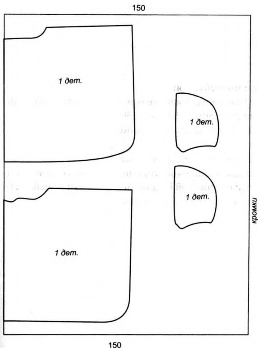
Схема раскладки полочки и капюшона
