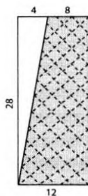
боковая часть для переда 2 дет.
