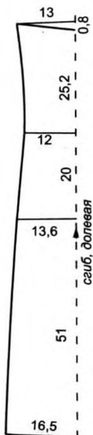
середина переда - 1 дет.
