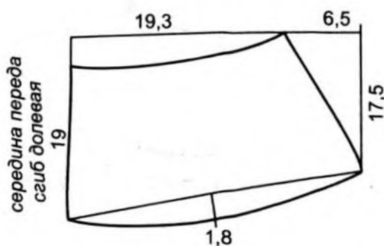
передняя кокетка юбки - 1 дет.
