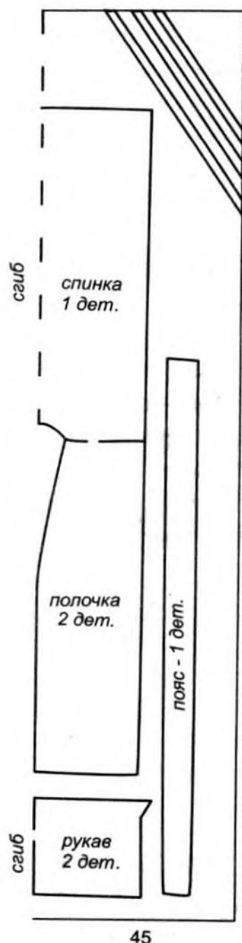
Схема раскладки при ширине 1,50 м
