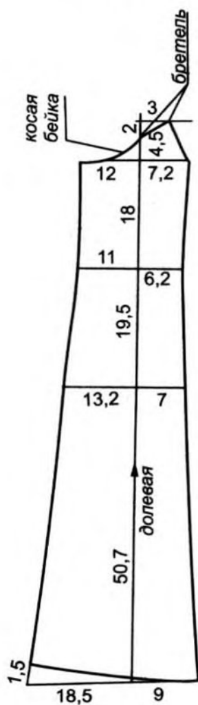
боковая часть переда - 2 дет.
