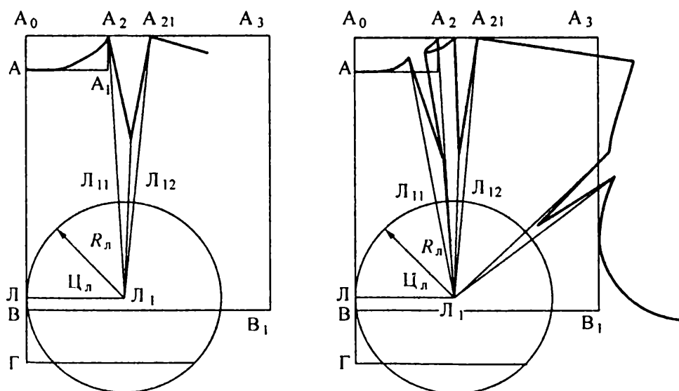
Рис. 6.3. Схема построения плечевой выточки и варианты ее перераспределения
