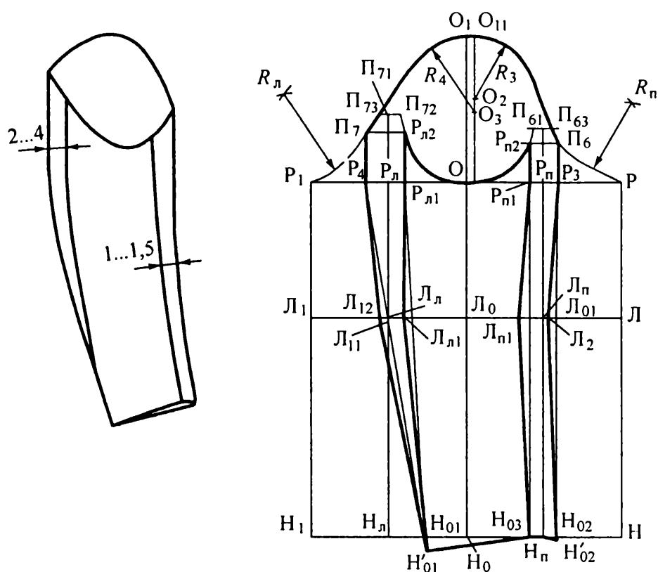
Рис. 6.14. Чертеж втачного двухшовного рукава, зауженного книзу
