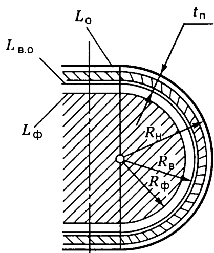
Рис. 5.10. Определение \Pi_{\text{п}} расчетным способом
