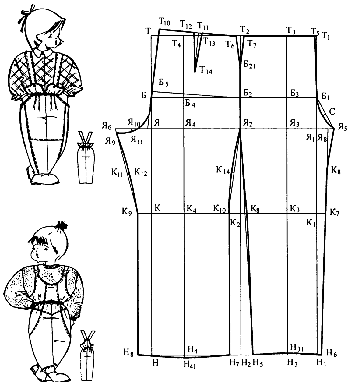
Рис. 12.3. Чертеж унифицированной ТБКО детских брюк
