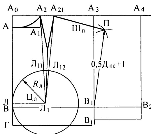
Рис. 6.4. Схема построения линии плечевого среза спинки
