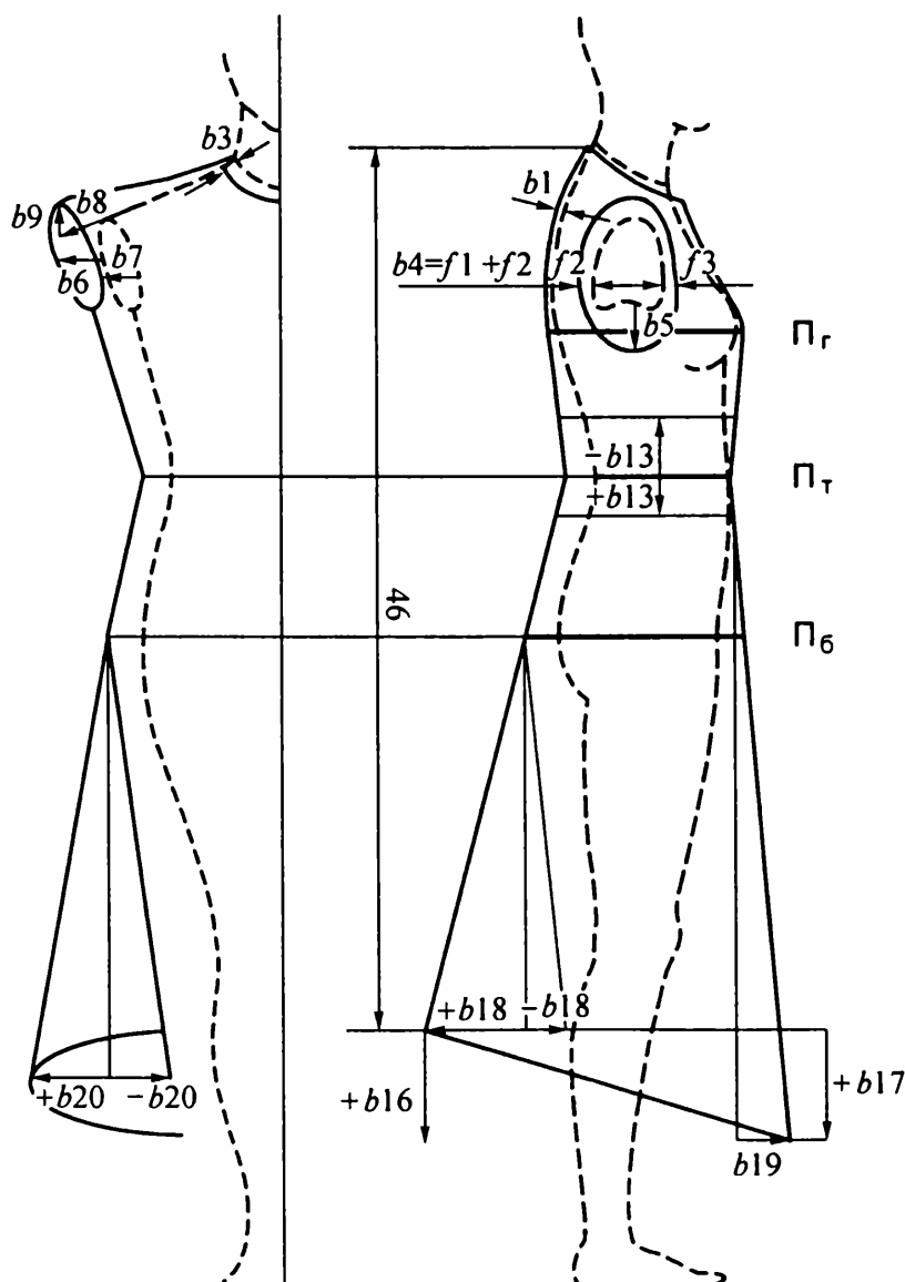
Рис. 5.13. Вариант задания формы в САПР СТАПРИМ
