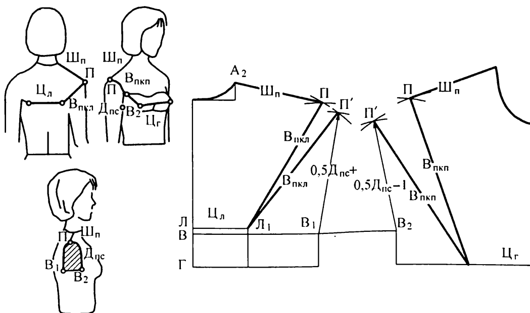
Рис. 5.25. Схема графического построения нагрудной и плечевой вытачек с использованием измерений Д_{пс} , В_{пкл} , В_{пкп} , Ш_п
