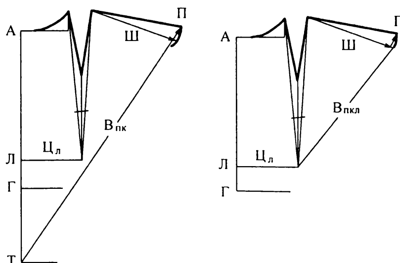
Рис. 5.20. Варианты построения плечевых срезов
