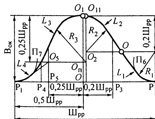
Рис. 5.18. Определение параметров рукава
