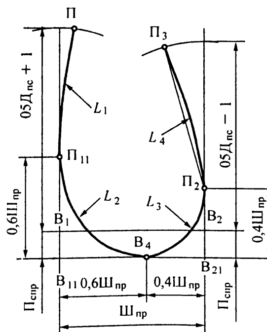
Рис. 5.17. Определение параметров проймы
