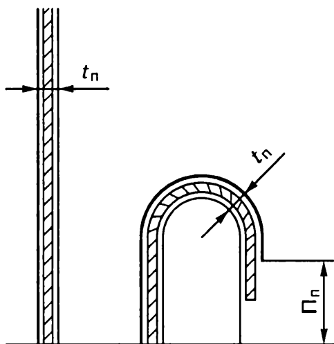
Рис. 5.9. Определение \Pi_{\text{п}} муляжным способом
