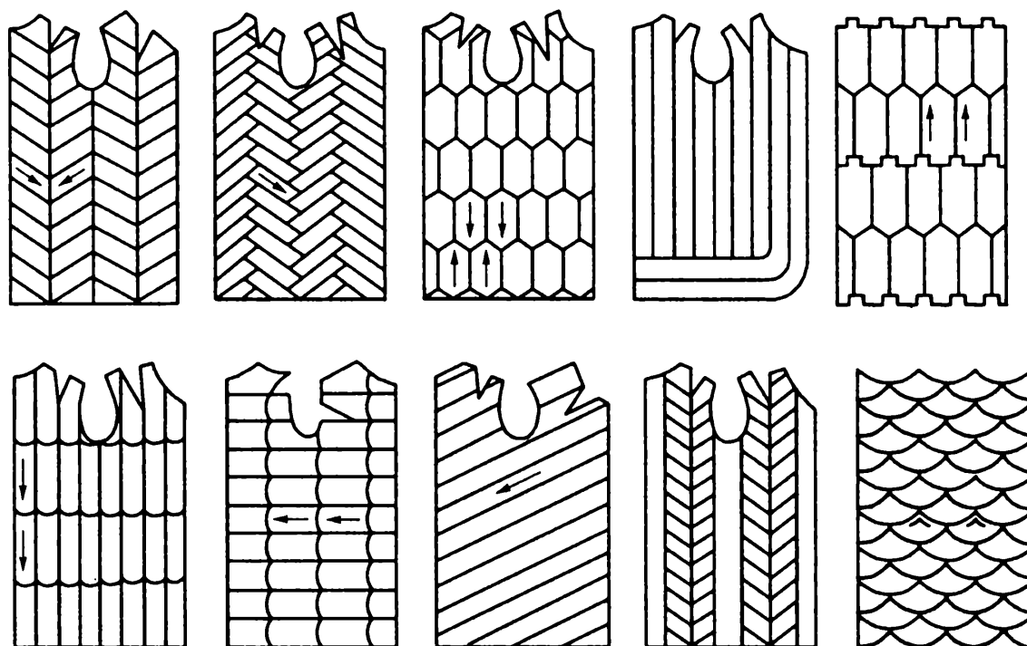
Рис. 13.6. Варианты объединения шкурок в пластины и детали
