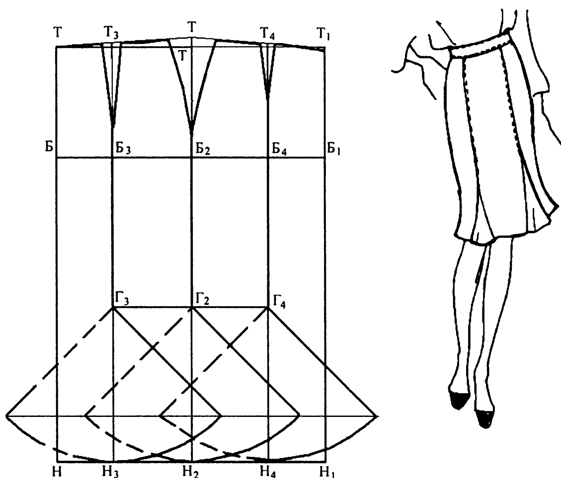
Рис. 10.8. Чертеж конструкции юбки «годе» на базе прямокроеной юбки
