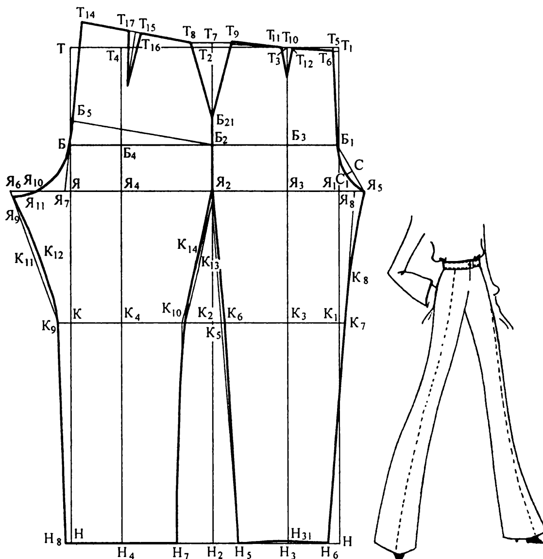
Рис. 10.10. Чертеж ТБКО женских длинных брюк
