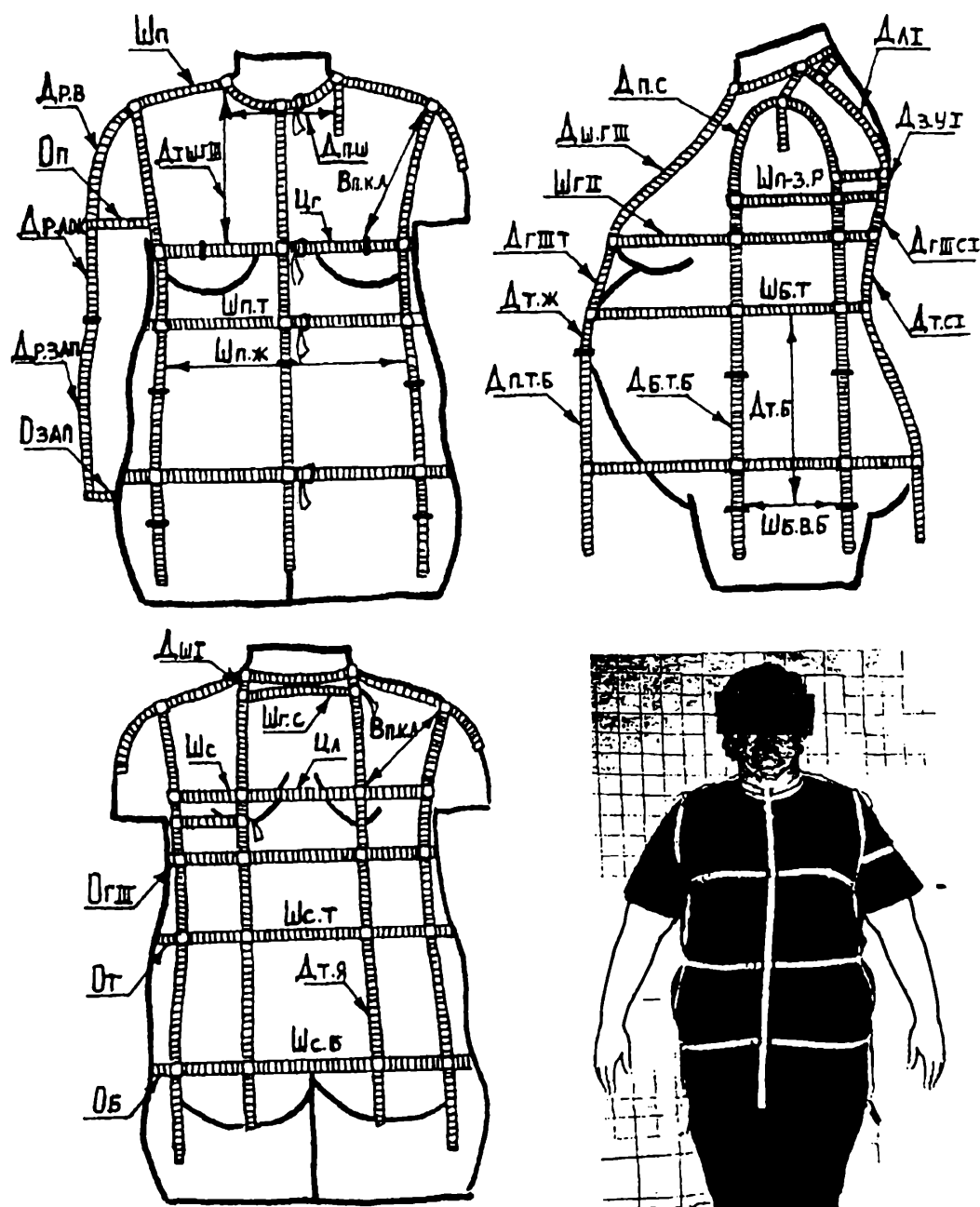
Рис. 5.7. Вид измерительного устройства по методике РосЗИТЛП
