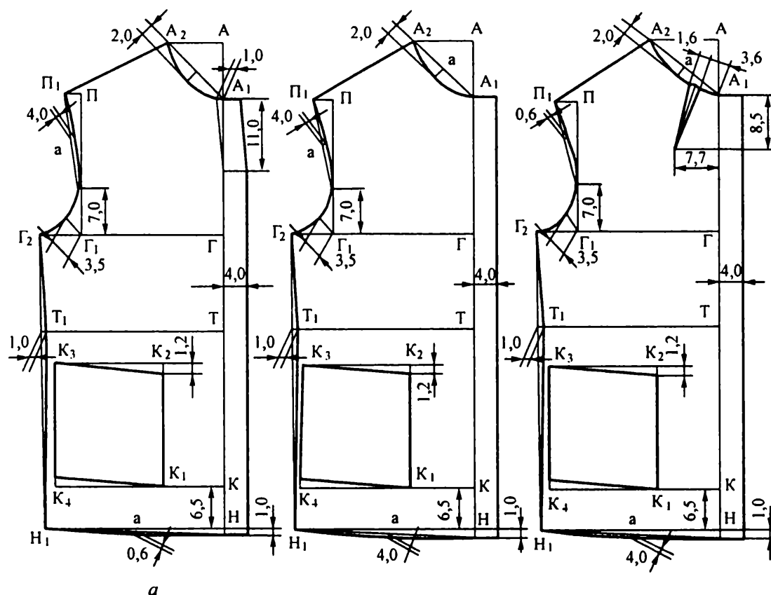
Рис. 14.3. Схема построения детали полочки мужской куртки
