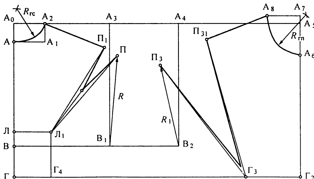
Рис. 6.6. Схема построения плечевой и нагрудной вытачек
