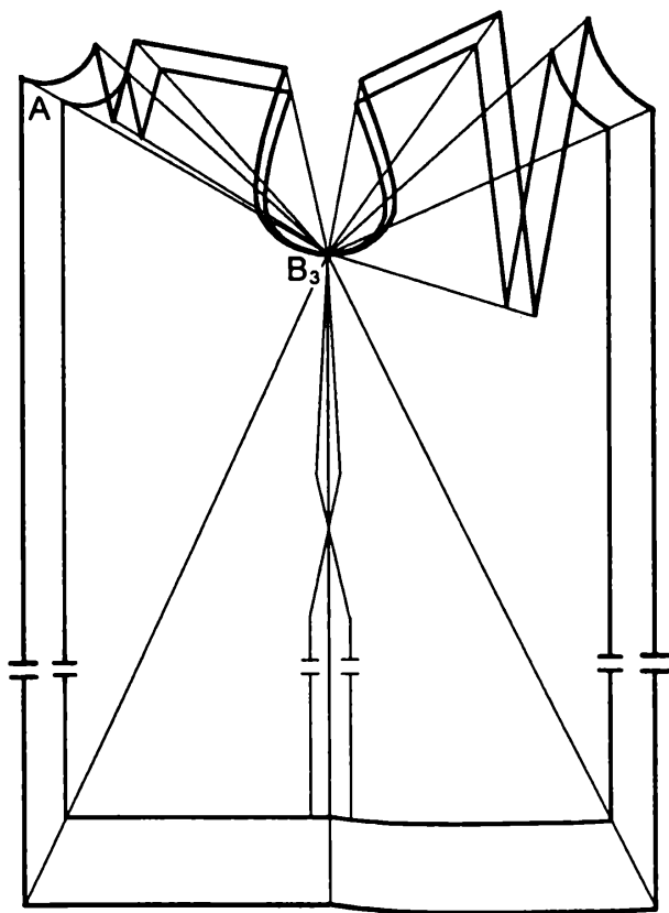
Рис. 5.12. Гомотетические преобразования с учетом толщины пакета
