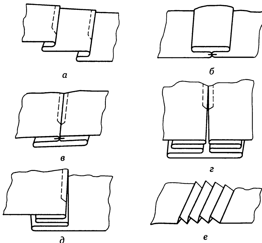
Рис. 3.21. Варианты складок
