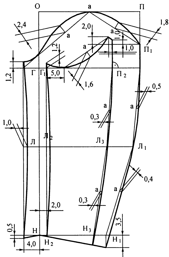
Рис. 14.5. Схема построения чертежа двухшовного рукава мужской куртки
