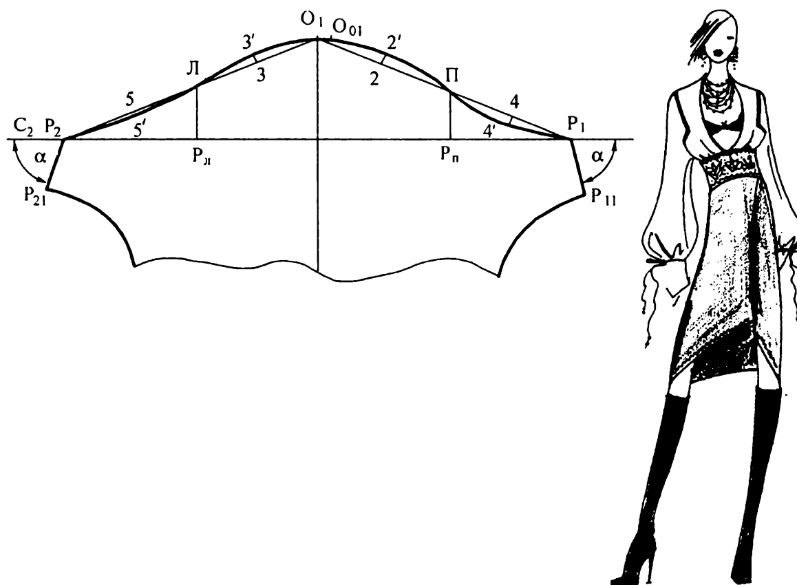
Рис.9.8. Чертеж конструкции втачного рукава рубашечного покроя в углубленную трапецевидную пройму
