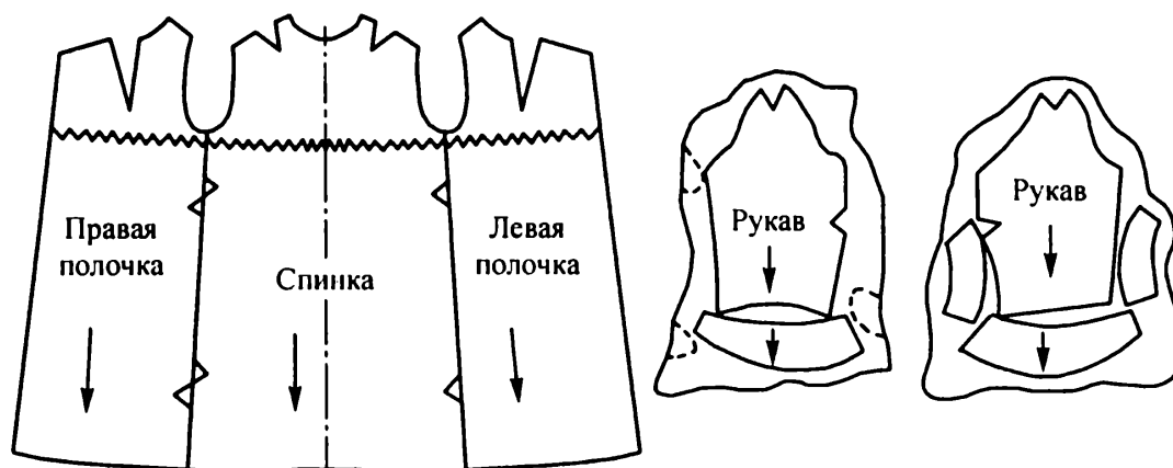
Рис. 13.9. Схема членения деталей изделия из крупных шкур
