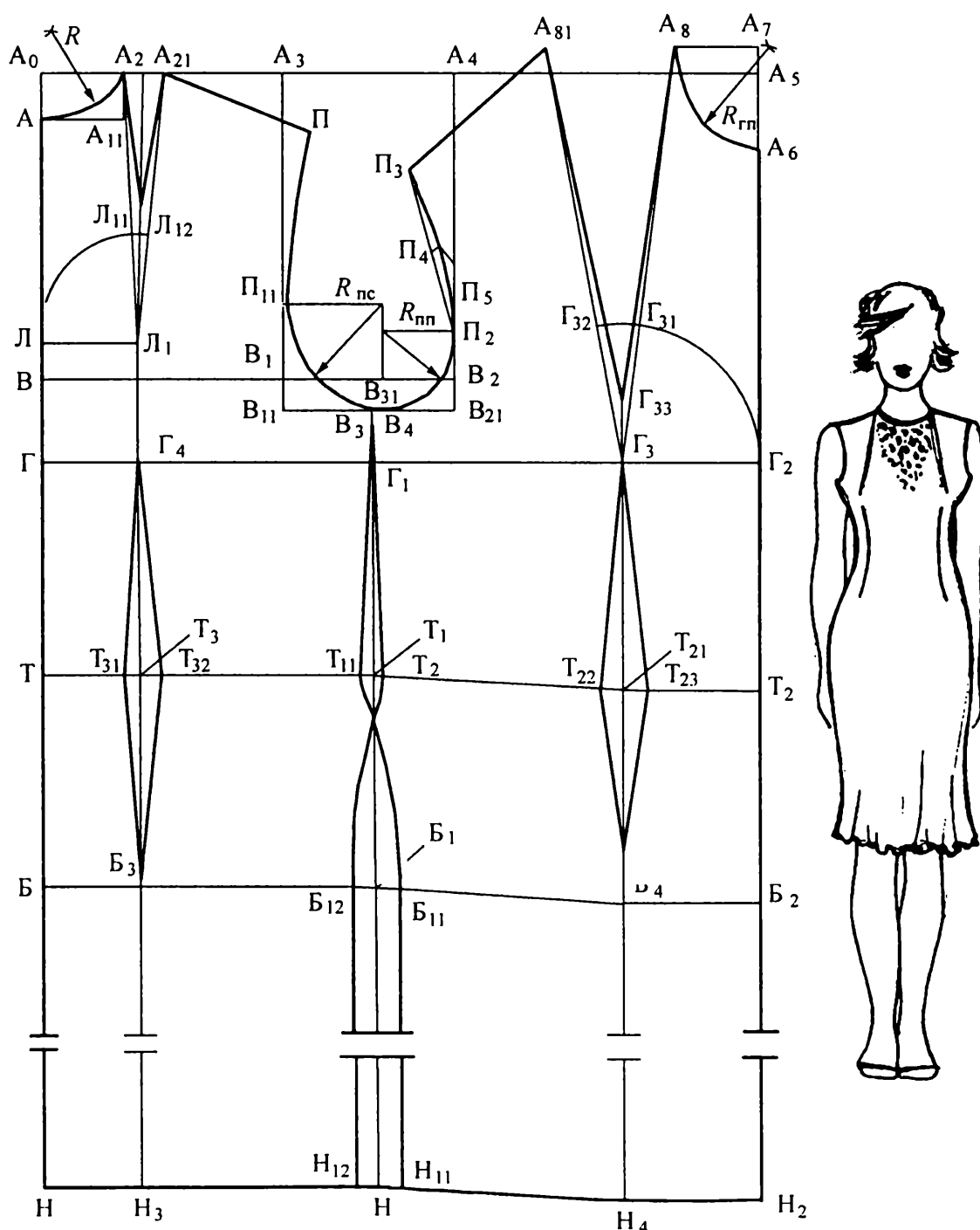
Рис. 6.8. Чертеж конструкции ТБКО плечевого женского изделия
