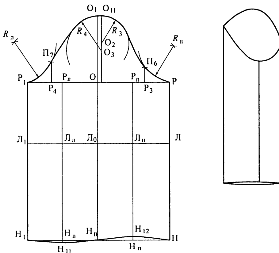
Рис. 6.11. Чертеж втачного одношовного прямого рукава
