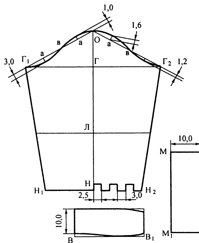
Рис. 14.4. Схема построения чертежа одношовного рукава, манжеты и нижнего воротника
