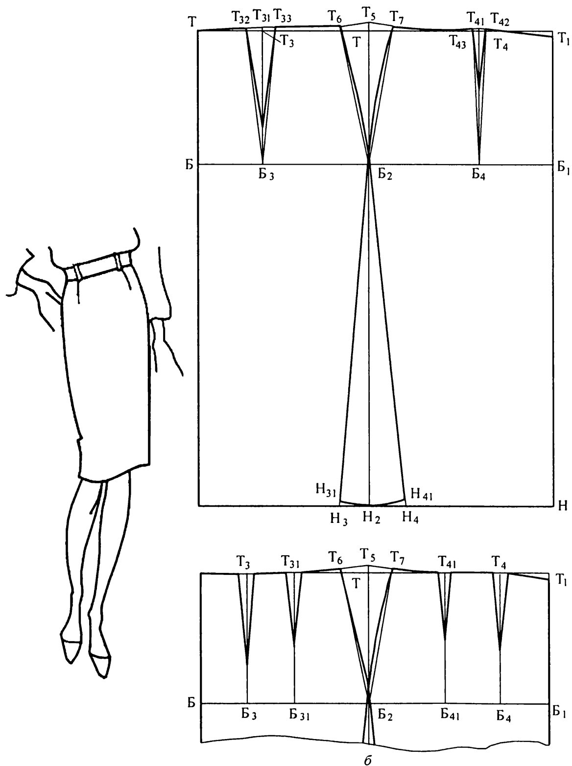
Рис. 10.4. Чертеж ТБКО прямокроеной юбки:
