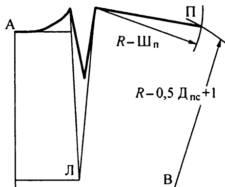
Рис. 5.22. Варианты построения плечевых срезов
