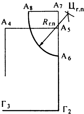
Рис. 6.2. Схема построения горловины спинки и переда
