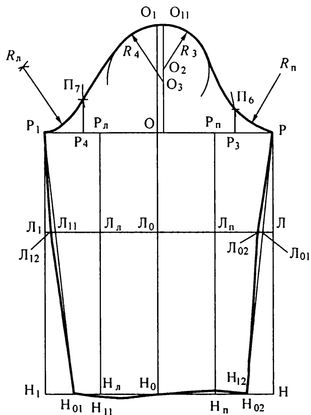
Рис. 6.12. Чертеж втачного одношовного рукава, зауженного книзу
