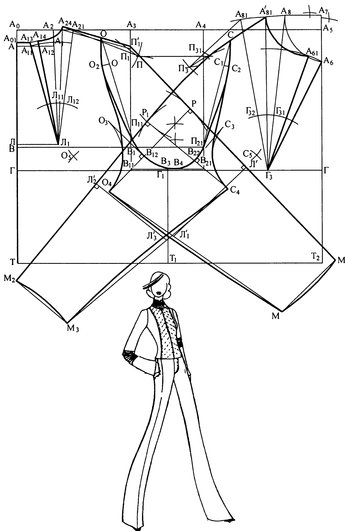
Рис. 8.7. Чертеж ТБКО плечевого изделия с рукавами покроя полуреглан
