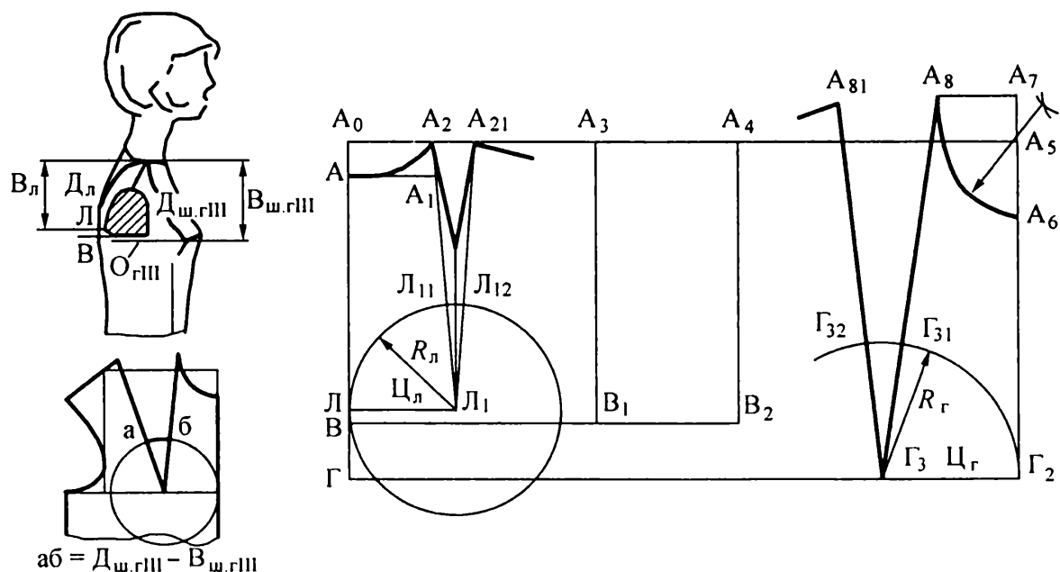
Рис. 5.26. Схема построения плечевой и нагрудной вытачек с использованием измерений B_{\text{л}} , B_{\text{ш.гIII}} , D_{\text{л}} , D_{\text{ш.гIII}}
