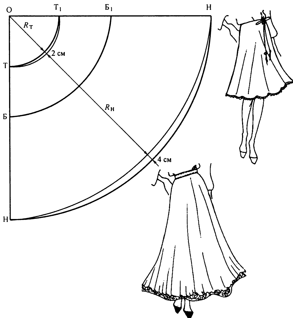
Рис. 10.9. Чертеж ТБКО юбки из \frac{1}{2} части круга
