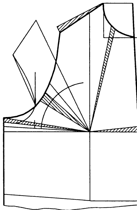
Рис. 11.7. Перераспределение нагрудной вытачки в трикотажном изделии
