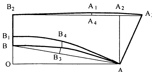
Рис. 6.15. Чертеж БК стояче-отложного воротника
