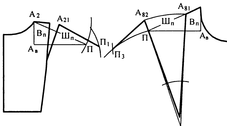
Рис. 5.21. Варианты построения плечевых срезов
