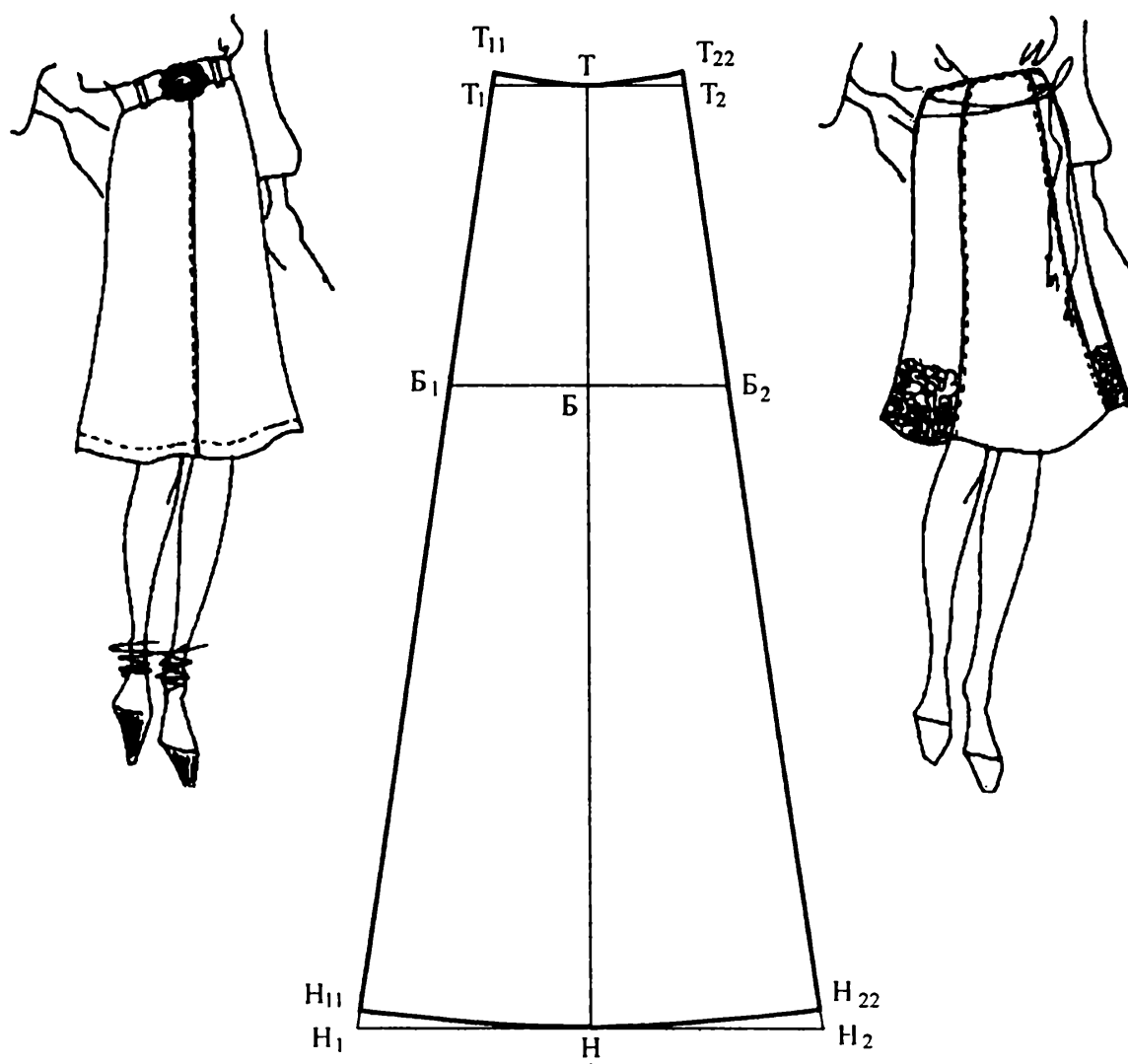
Рис. 10.5. Чертеж клина
