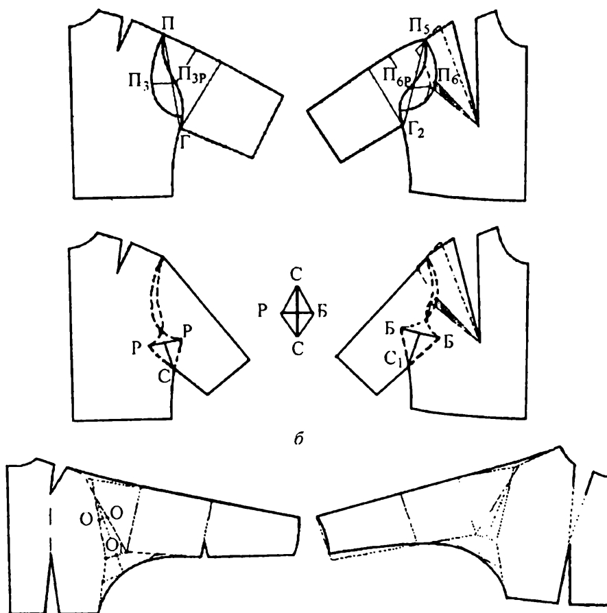
Рис. 7.4. Схемы графического построения чертежей деталей цельнокроеного рукава:
