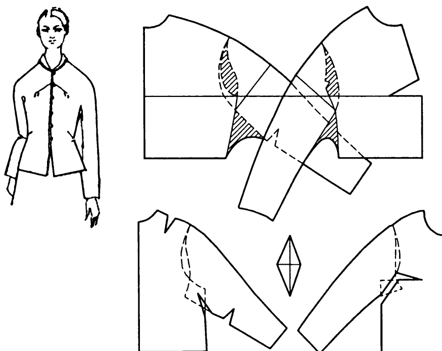
Рис. 4.8. Схема конструкции изделия с цельновыкроенными рукавами
