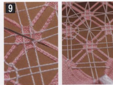
次のredondoの中央に裏から針を出し、隣に表から入れ、木杵の向きを90°変えてredondoを作る
