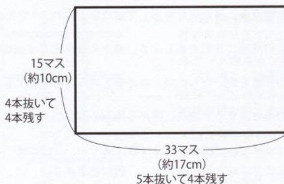
寸法図
