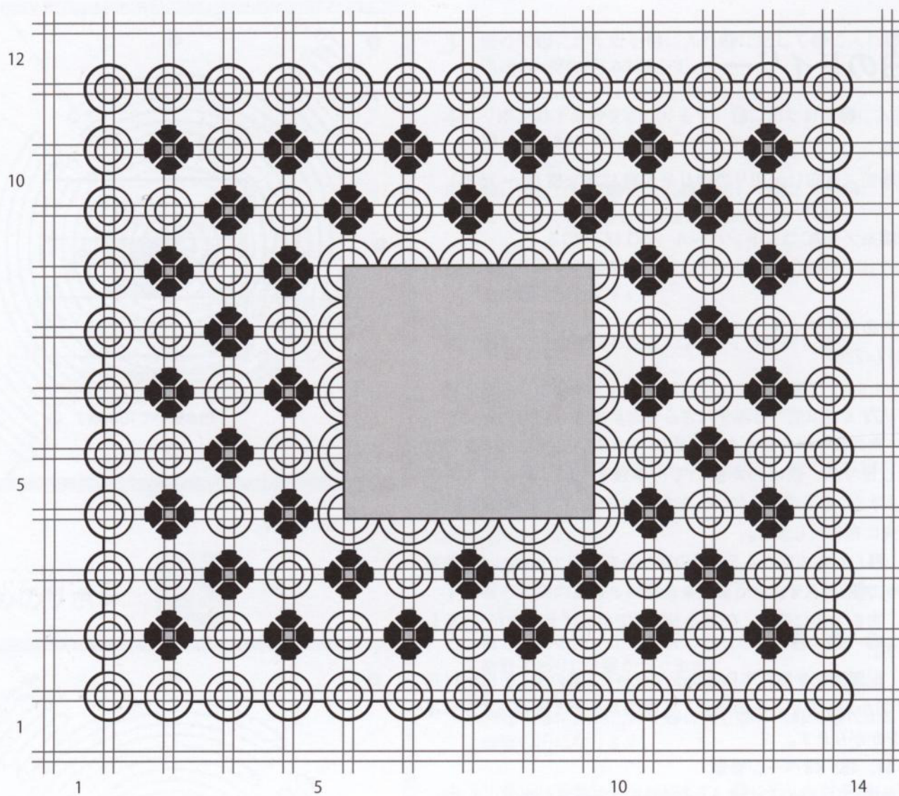
配置図
