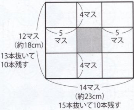
寸法図
