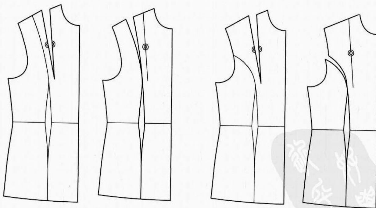
(6) 省道转移的方法示意图
