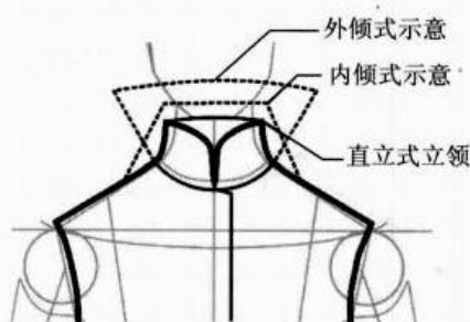
▲图 29 三种基本类型的立领样式示意图
