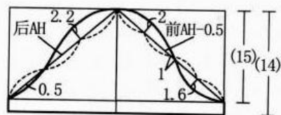
►袖片
