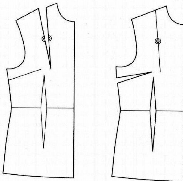
腋下省转移
