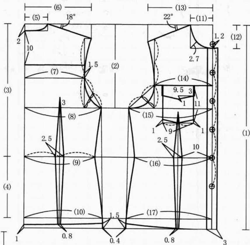
►主身片
