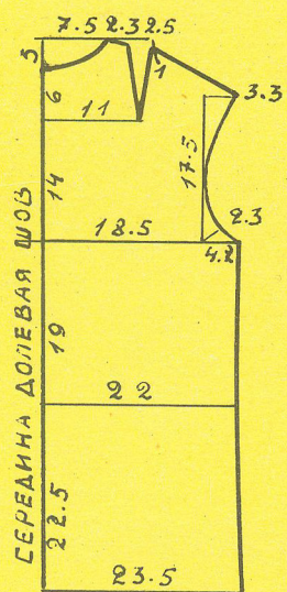
СПИНКА БЛУЗЫ 2 ДЕТ.
