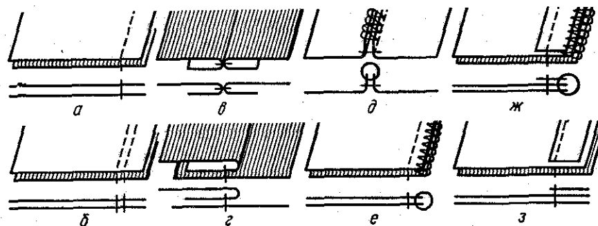
Рис. 51. Стачные швы:
