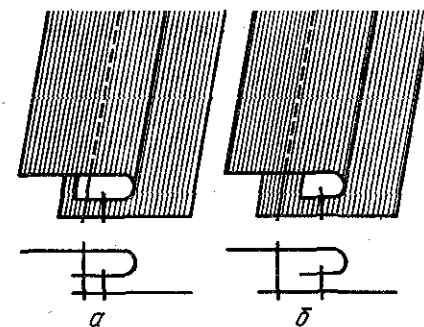
Рис. 53. Настрочные швы: а — с двумя открытыми срезами; б — с одним закрытым срезом.
