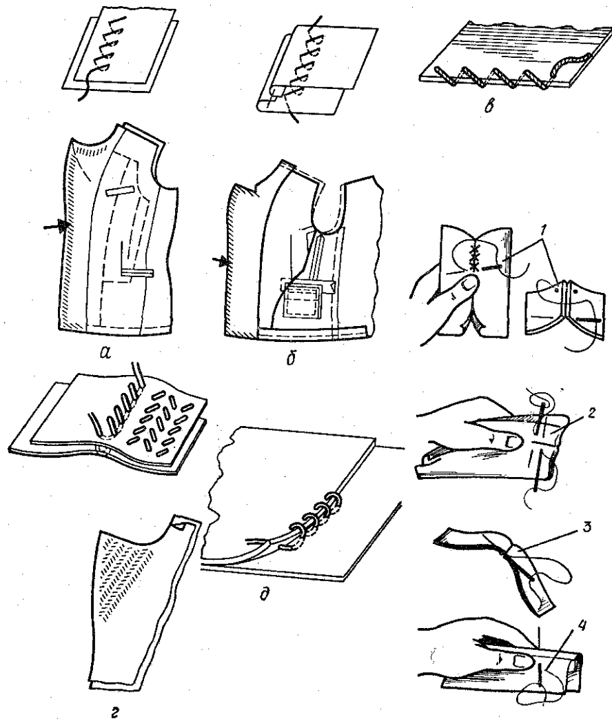
Рис. 31. Строчки, образованные с помощью косых стежков: а — наметочная; б — выметочная; в — обметочная; г — стегальная; д — подшивочная; е — для незаметного скрепления деталей: 1—3 — штуковка, 4 — рас- пошивка.
