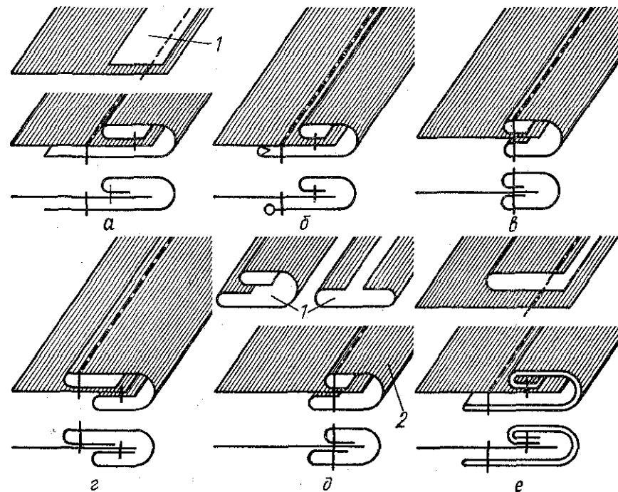
Рис. 63. Окантовочные швы:
