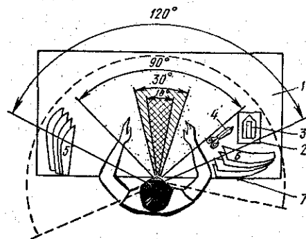
Рис. 5. Поле зрения утюжильщицы при организации рабочего места: 1 — крышка стола; 2 — подставка для утюга; 3 — утюг; 4 — ножницы; 5, 6 — полуфабрикаты до и после выполнения операций; 7 — пульверизатор.
