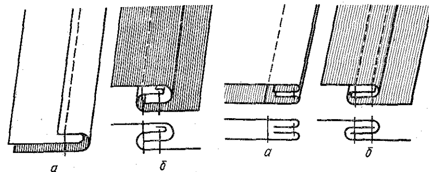
Рис. 58. Запошивочные швы: а, б — стадии получения шва.
