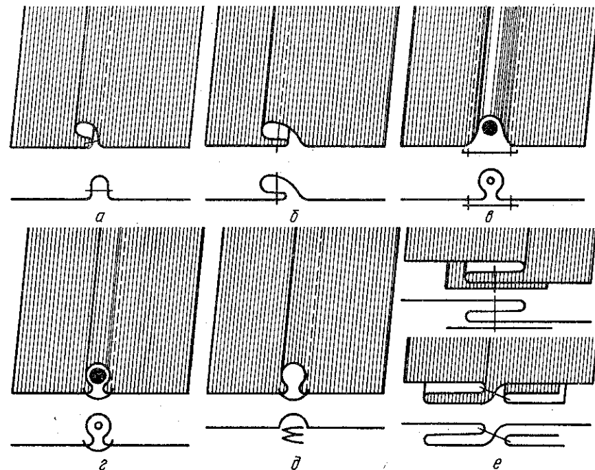
Рис. 66. Рельефные швы:
