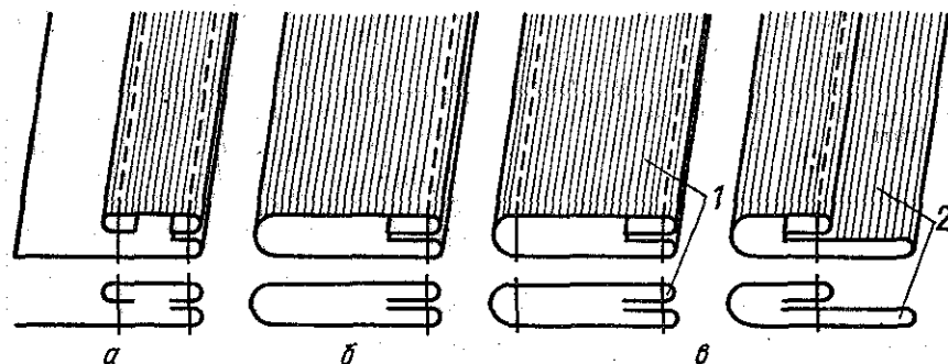
Рис. 55. Примеры использования накладных швов: а — настрачивание отделочных беек по краю детали; б — обработка пояса; а — обработка бретелей; 1 — с расположением шва по краю, 2 — с расположением шва посередине.
