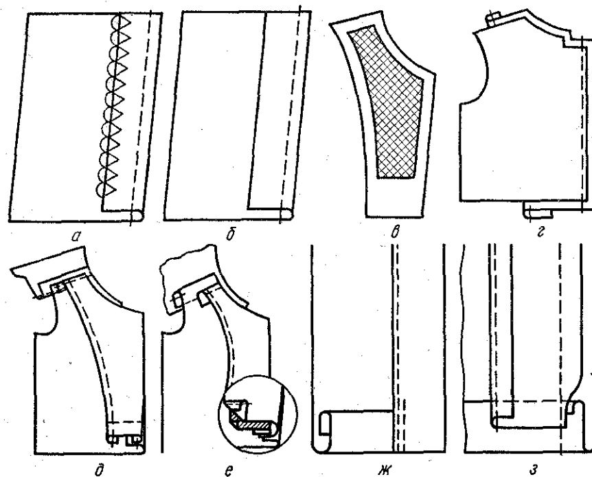
Рис. 80. Обработка бортов подбортами.
