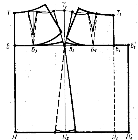
Рис. 21. Техническое моделирование формы юбки.
