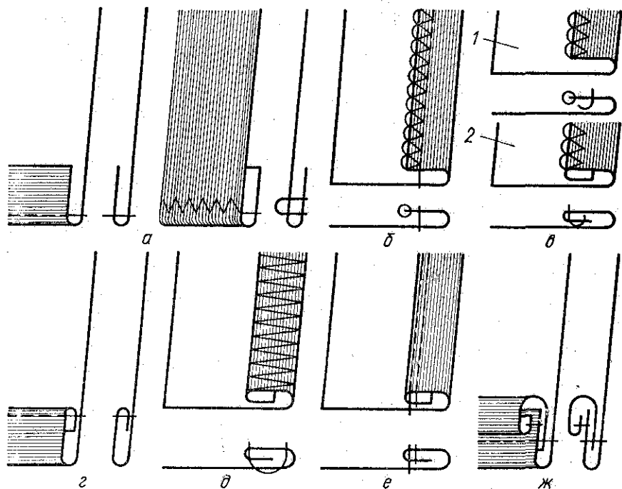
Рис. 62. Швы вподгибку:
