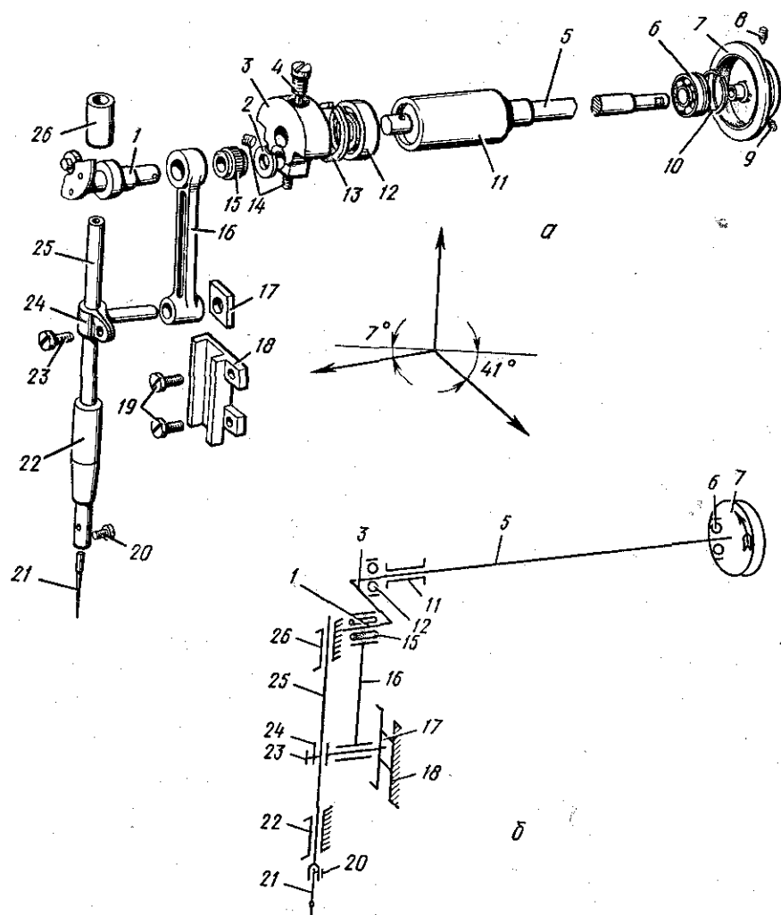
Рис. 42. Механизм иглы машины 97-А кл. ОЗЛМ: а — конструктивная схема; б — структурная схема.
