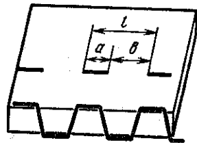
Рис. 27. Размеры прямого стежка:
