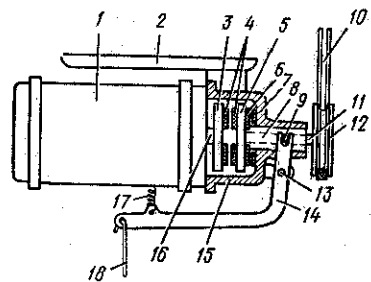
Рис. 43. Схема индивидуального электропривода.
