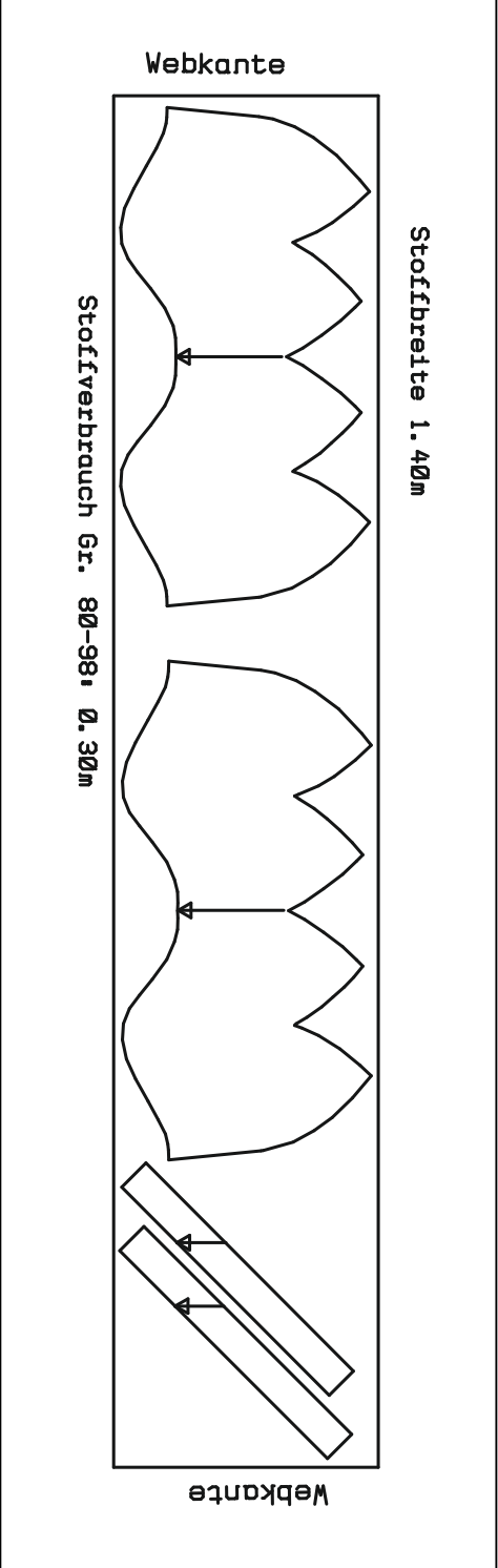
Zuschneideplan Gr. 80-98
