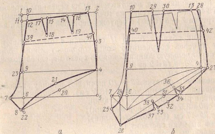
Рис. 33. Чертеж плавок
