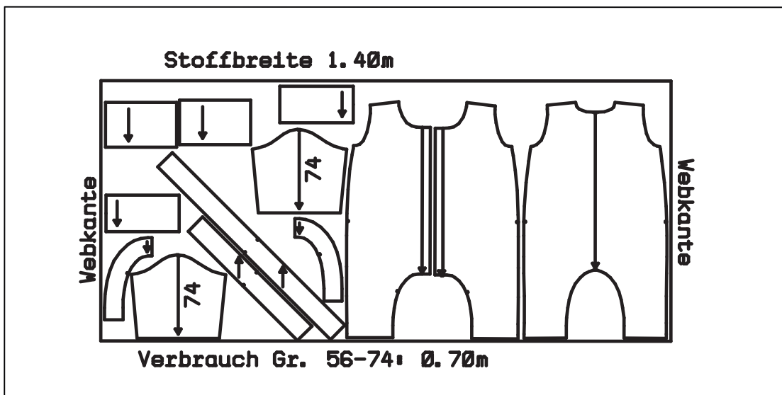
Zuschneideplan Gr. 56-74
