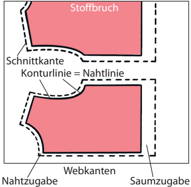
Nahtzugabe Webkanten Saumzugabe
