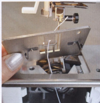
3. Gummifaden durch den Greiferraum
