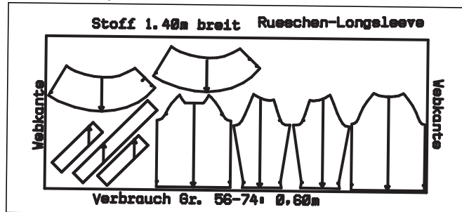
Zuschneideplan Gr. 56-74
