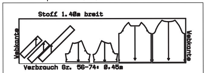
Zuschneideplan Gr. 56-74
