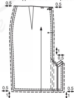
Рис. 9 Бочок, цельнокроеный с подкладкой кармана
