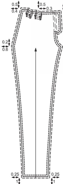
Рис. 8 Передняя половинка брюк
