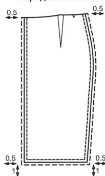
Рис. 11 Переднее полотнище юбки
