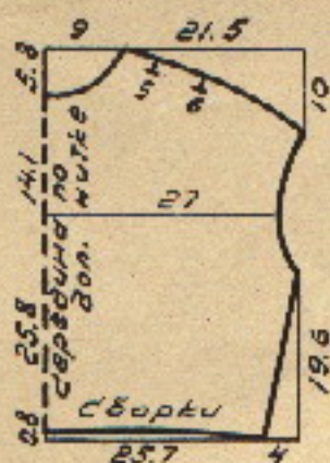
Спинка лифа
