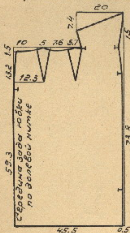
правое полотно
