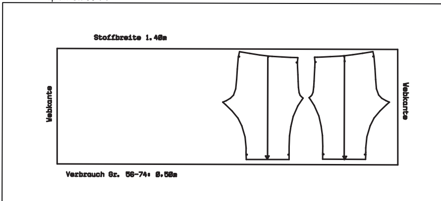
Zuschneideplan Gr. 56-74
