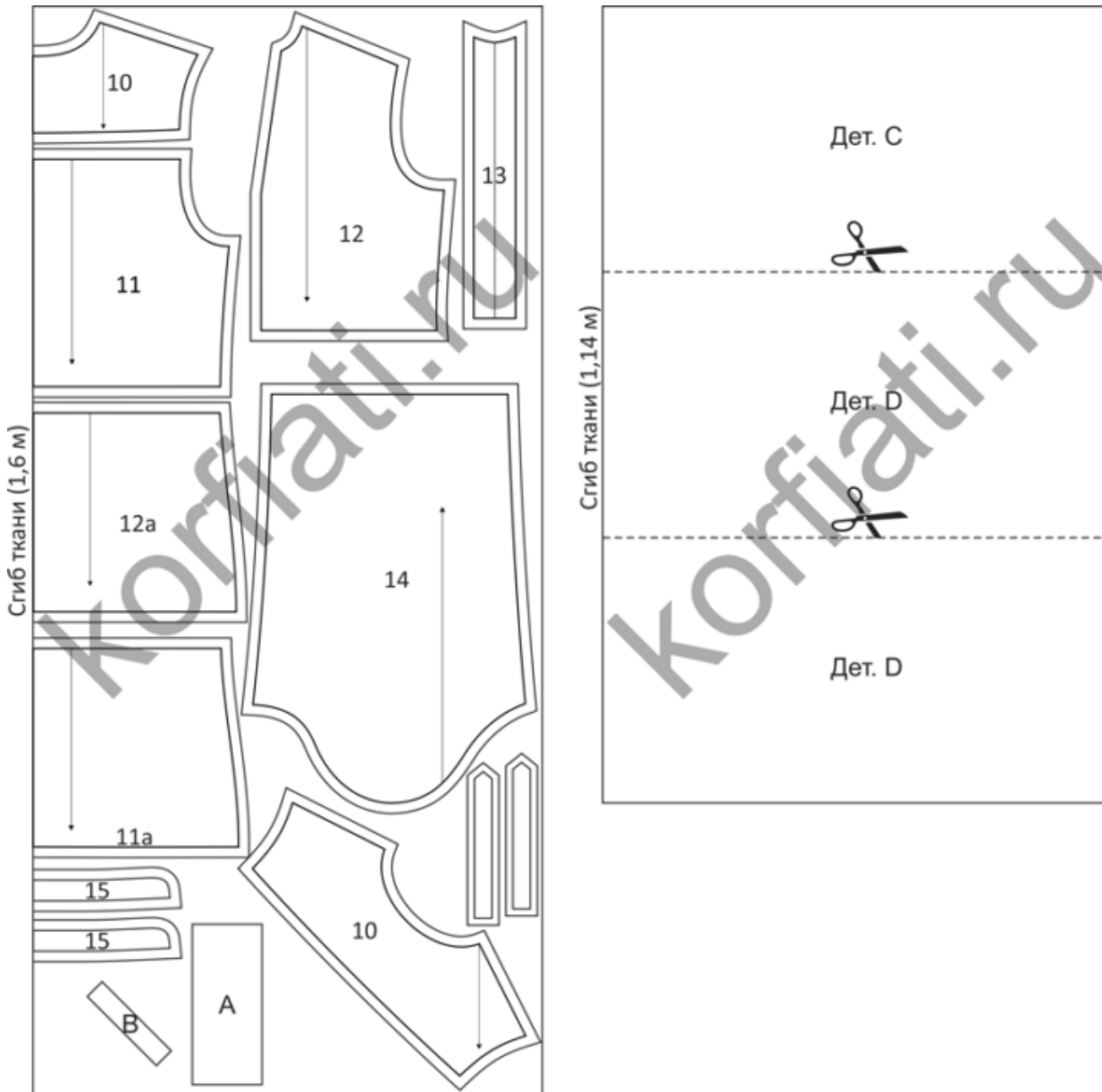
Рис. 4. Раскладка деталей платья на материале
