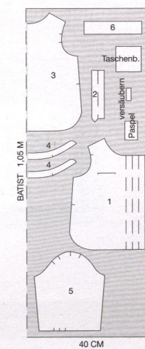
ZUSCHNEIDEPLAN
