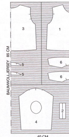
ZUSCHNEIDEPLAN
