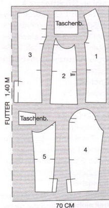
Bogen 4. Bogenseite B. Schwarze Schnittmusterlinien. Größen: 36 - 40 - 44
