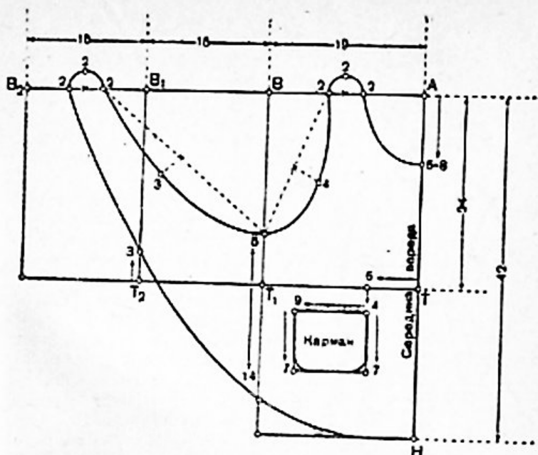
Рис. 64. Чертеж выкройки детского фартука.
