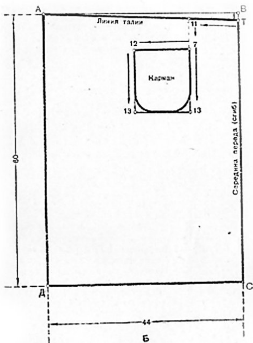
Рис. 308 б. Чертеж выкройки нижней части фартука
