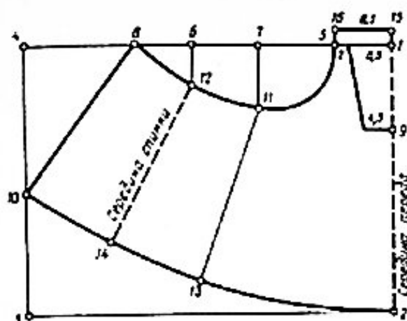
Рис. 197. Чертеж передника, расширенного книзу (модель 4)
