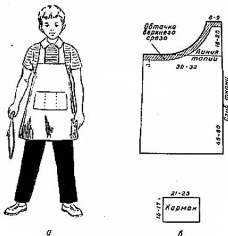
Рис. 160. Рабочий фартук для уроков труда: а — общий вид; б — раскрой.
