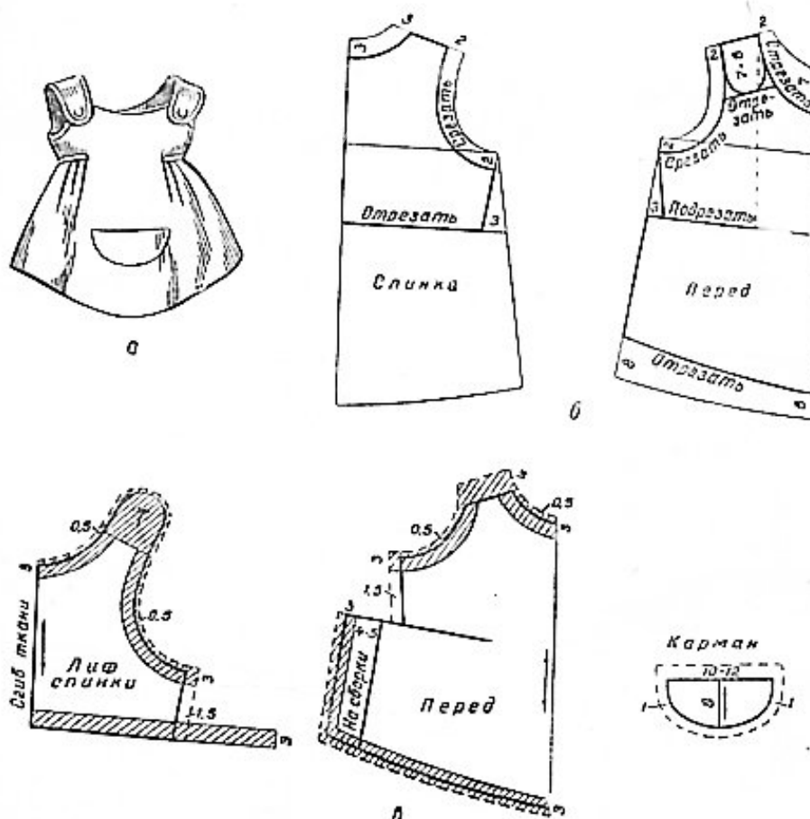
Рис. 70. Передник с подрезом от бокового среза: а — общий вид; б — подготовка выкройки к раскрою; в — раскрой.
