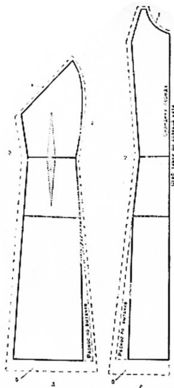
Рис. 310 д, е. Разработка фартука: д, е — раскладки деталей выкройки перед и спинки с припусками на швы.
