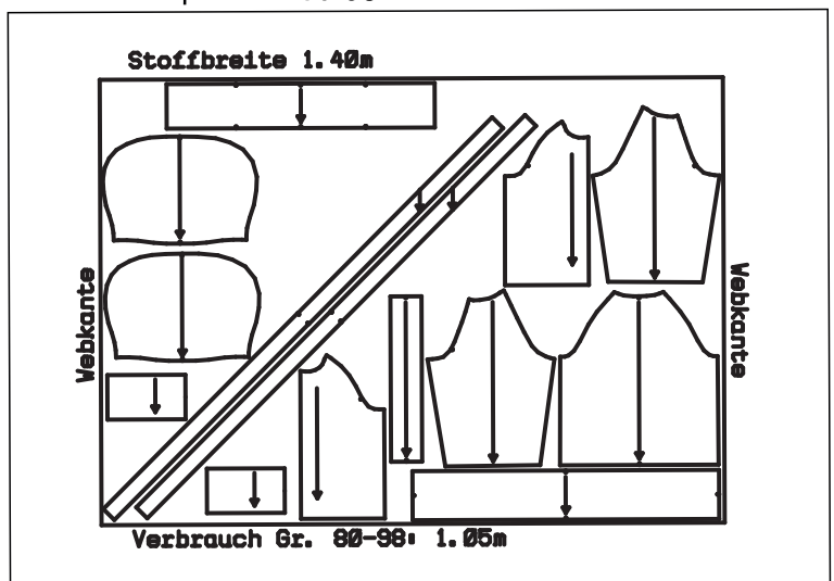
Zuschneideplan Gr. 80-98
