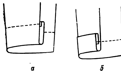
Рис. 28. Обработка рукавов с отворотами
