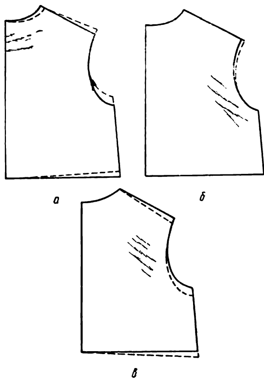
Рис. 17. Исправление недостатков спинки изделия
