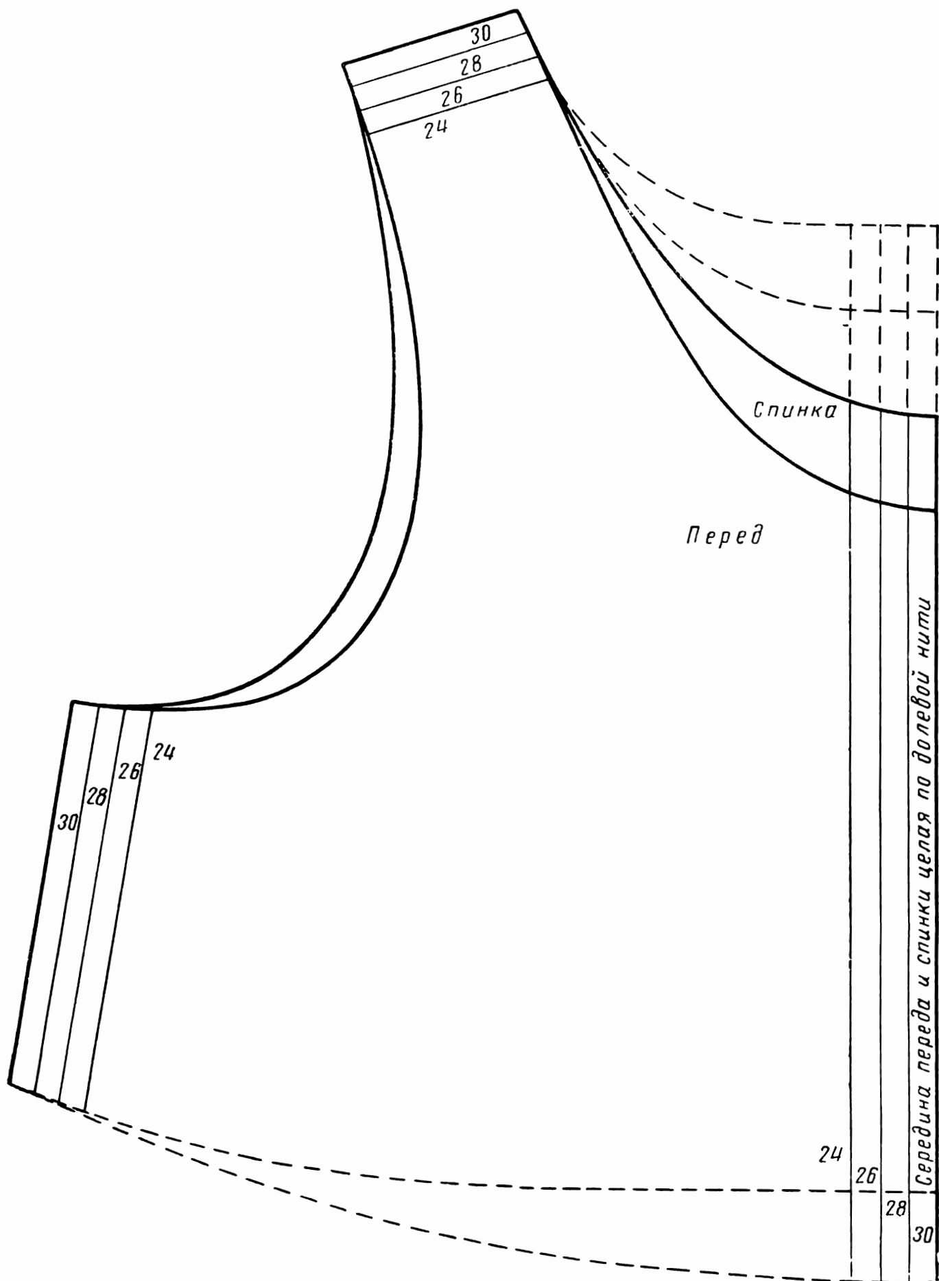
Рис. 49. Выкройка майки
