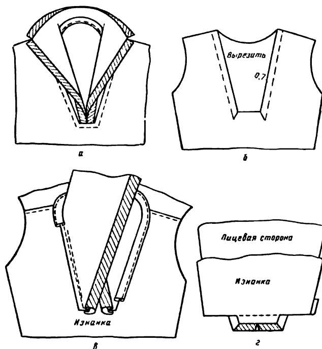
Рис. 40. Соединение матросского воротника с горловиной изделия
