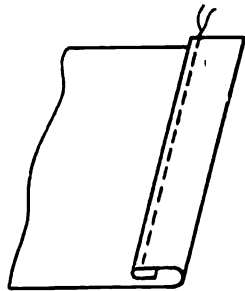
Рис. 12. Шов вподгибку с закрытым срезом
