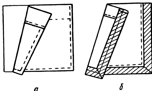
Рис. 23. Обработка накладного кармана: а — с подгибом обрезных краев; б — с обтачкой
