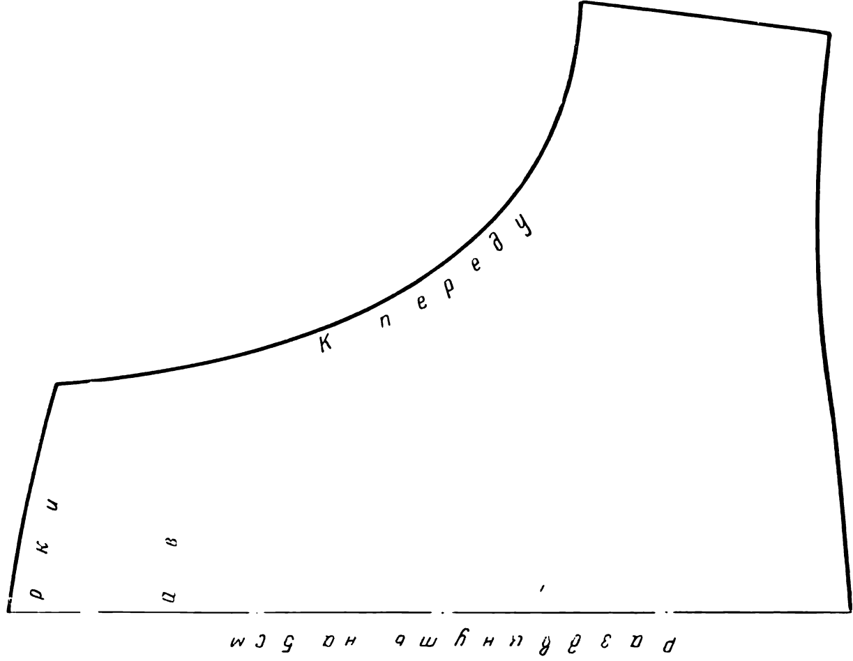
Рис. 58. Выкройка рукава сорочки с круглой кокеткой
