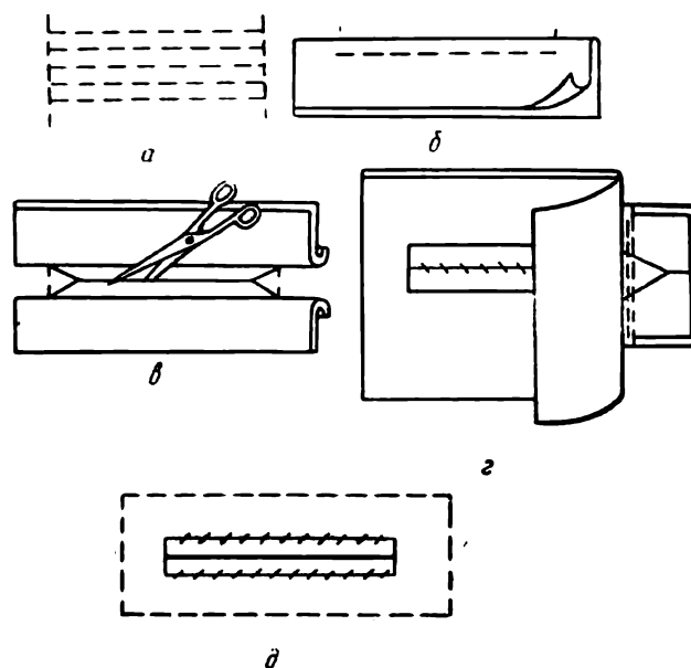
Рис. 36. Обработка петель двумя обтачками
