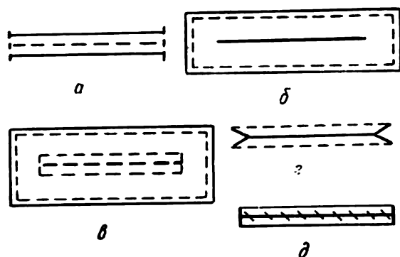
Рис. 35. Обработка петель одной обтачкой
