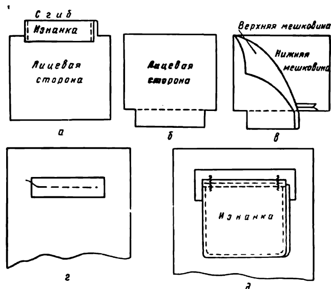
Рис. 25. Обработка прорезного кармана с листочкой
