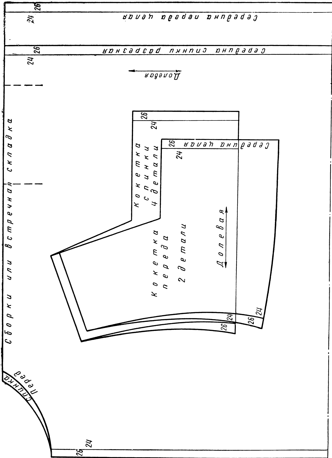
Рис. 66. Выкройка фартука на кокетке
