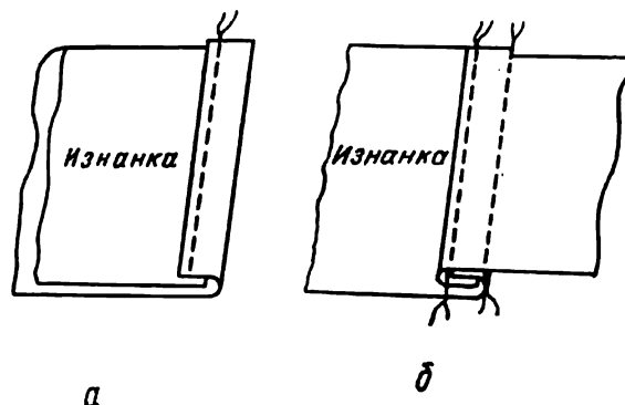
Рис. 11. Запошивочный, или бельевой шов: а — стачивание; б — настрачивание
