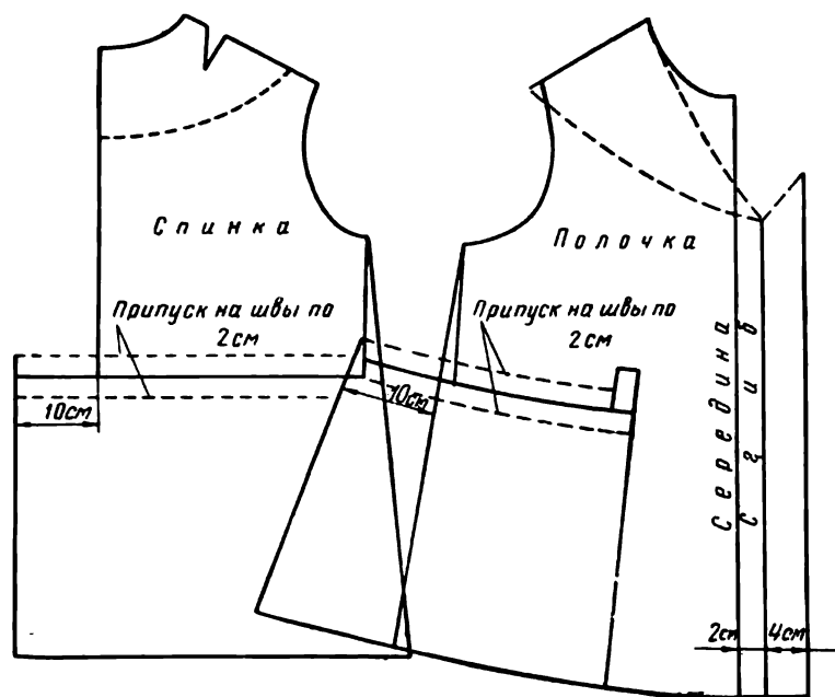
Рис. 114. Подготовка выкройки платья с подрезами по линии талии
