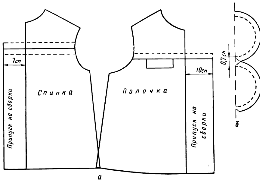
Рис. 101. Подготовка выкройки платья на прямой кокетке
