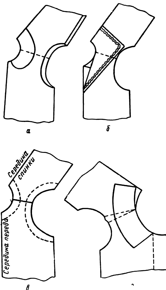
Рис. 19. Выкраивание отложных воротников и обтачек горловины
