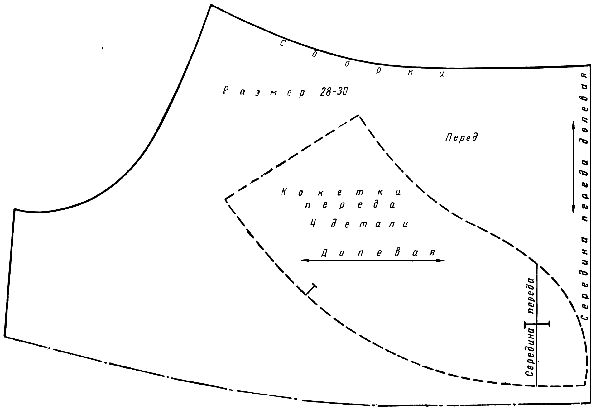
Рис. 56. Выкройка переда сорочки с круглой кокеткой
