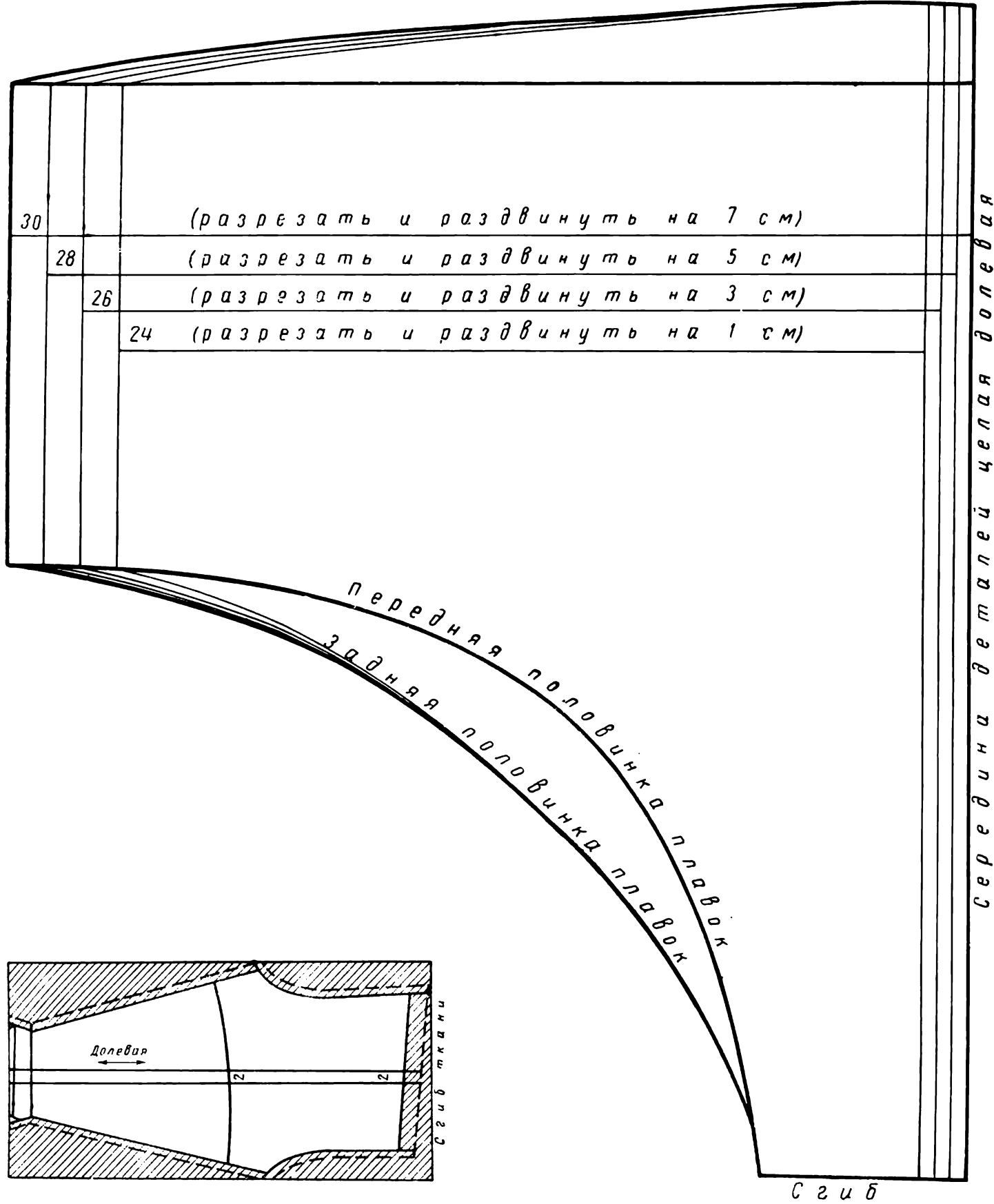
Рис. 47. Раскрой длинных спортивных брюк по выкройке трусов
