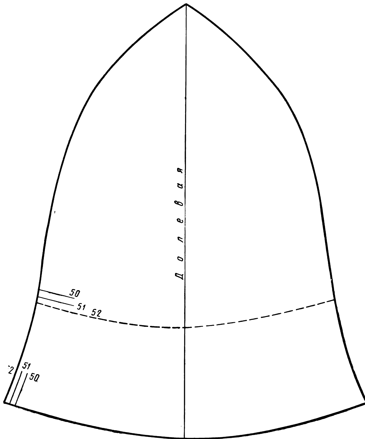
Рис. 85. Выкройка панамы
