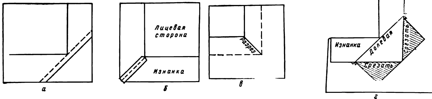
Рис. 44. Обработка внешних и внутренних углов на деталях изделия
