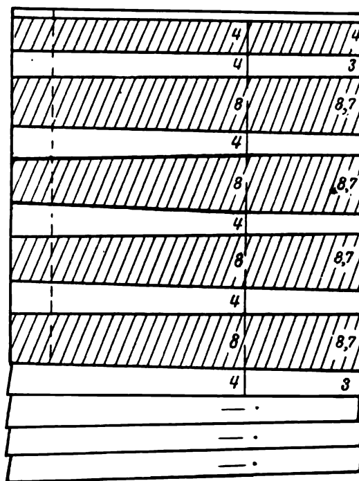
Рис. 76. Выполнение складок на юбке
