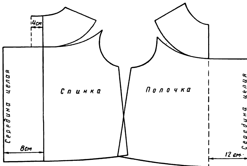
Рис. 104. Подготовка выкройки платья на круглой кокетке
