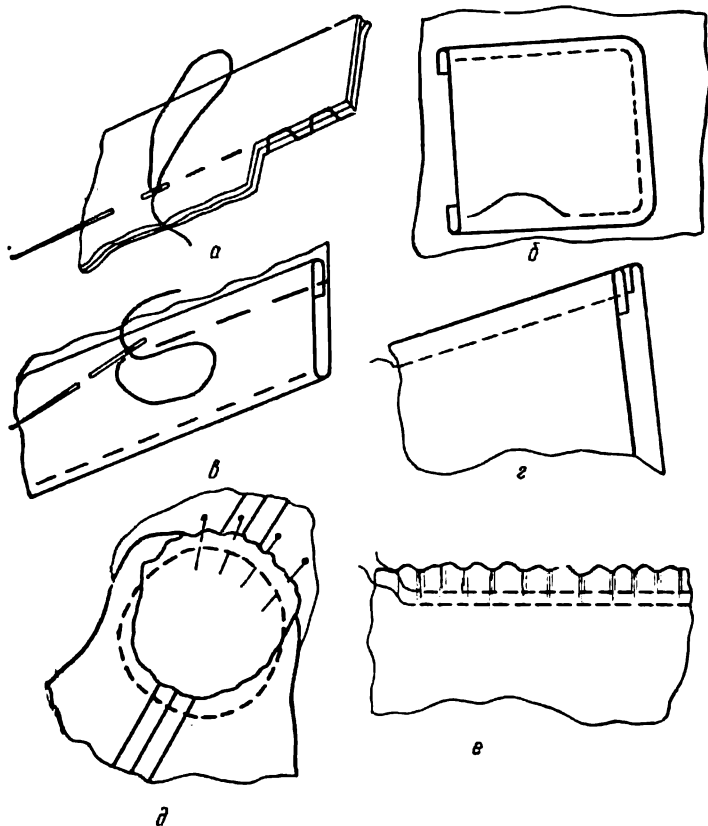
Рис. 1. Сметочные прямые стежки и выполняемые ими работы: а — сметывание; б — наметывание; в — заметывание; г — выметывание; д — вметывание; е — выполнение сборок
