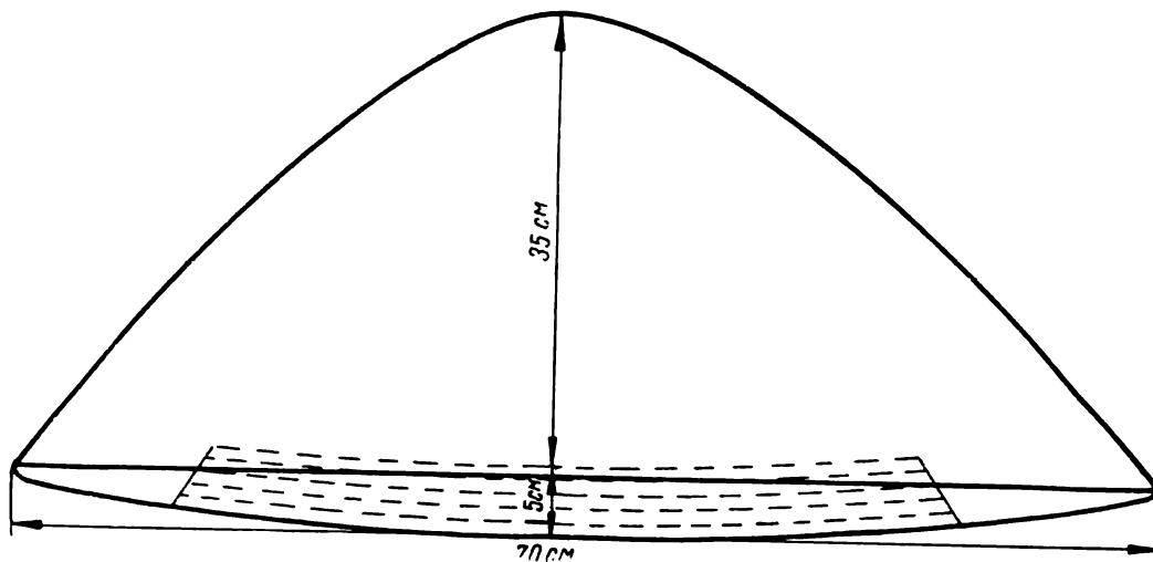
Рис. 81. Выкройка шапочки-косыпки
