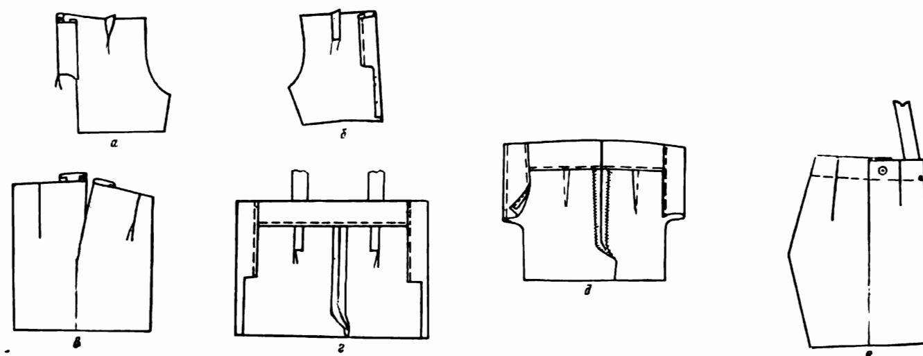
Рис. 78. Обработка брюк
