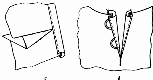
Рис. 30. Обработка разреза переда одной планкой: а — притачивание и настрачивание планки; б — застрачивание складочки в конце разреза переда
