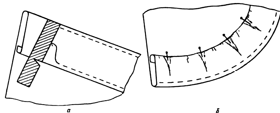
Рис. 43. Обработка низа изделия
