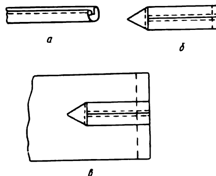
Рис. 39. Петли из ткани
