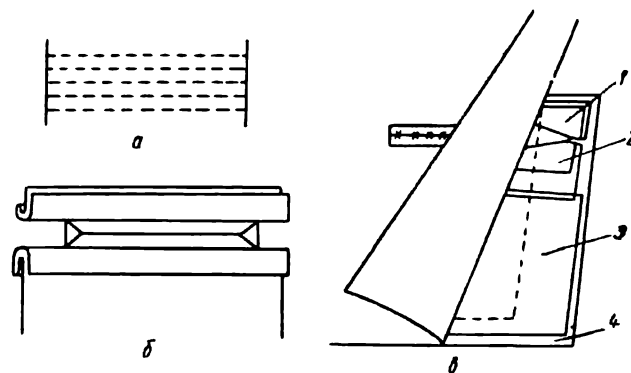
Рис. 24. Обработка прорезного кармана в рамку
