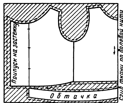
Рис. 54. Раскладка на ткани выкройки лифчика
