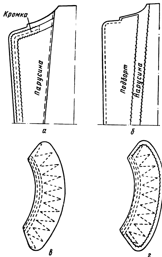
Рис. 77. Обработка бортов и воротника пальто
