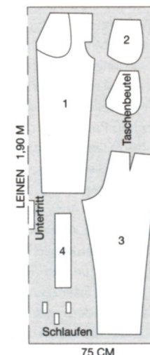
ZUSCHNEIDEPLAN
