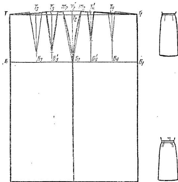
Рис. 31. Изменение положения вытакс с целью зрительного расширения и уплощения фигуры
