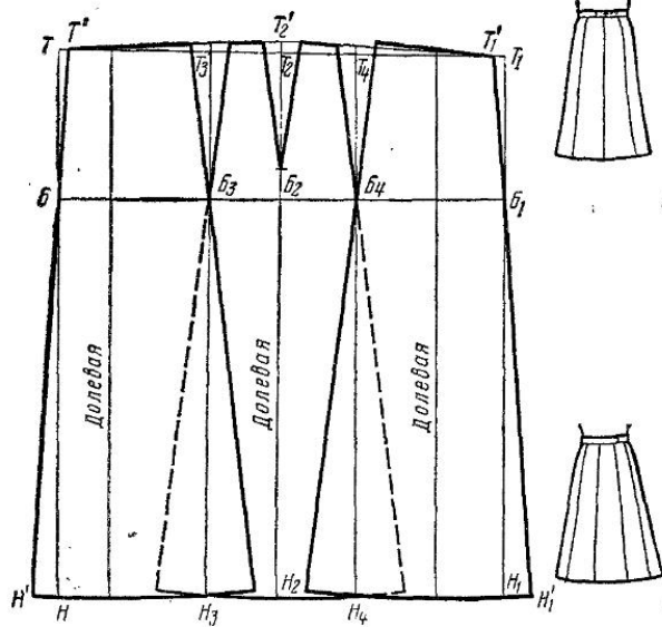
Рис. 11. Чертеж второго варианта шестিশовой юбки
