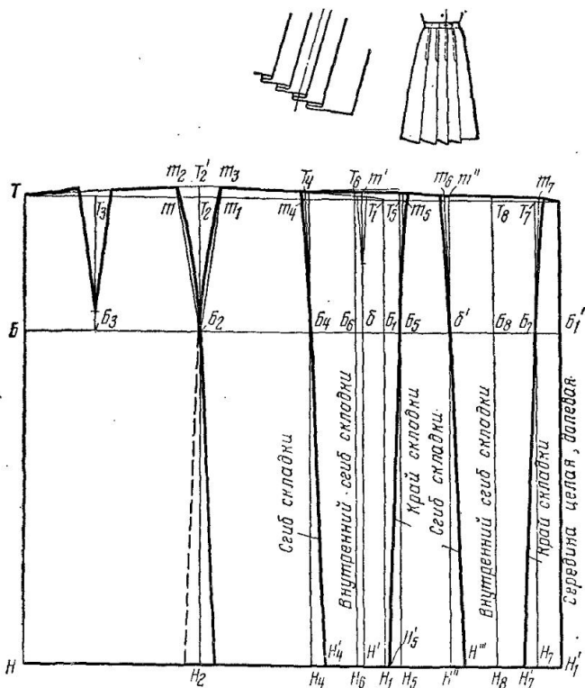
Рис. 25. Чертеж прямой юбки с четырьмя односторонними складками спереди
