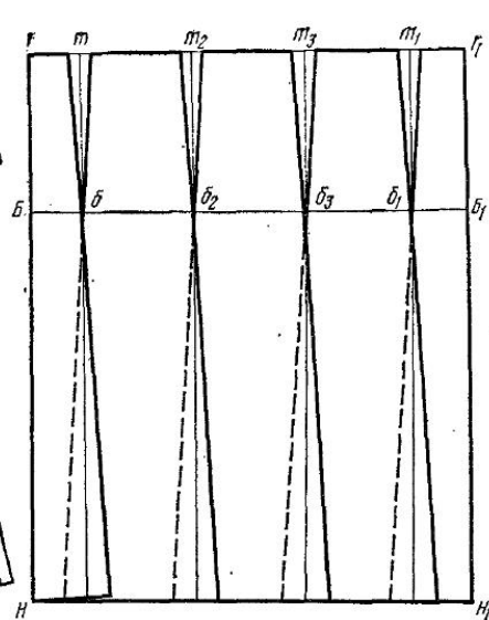
Рис. 12. Чертеж восьмিশовой юбки
