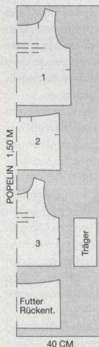
ZUSCHNEIDEPLAN
