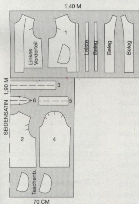
ZUSCHNEIDEPLAN
