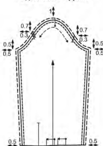
Рис. 4 Одношовный рукав
