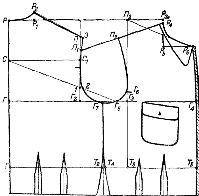
Рис. 74. Чертеж блузы конькобежного костюма
