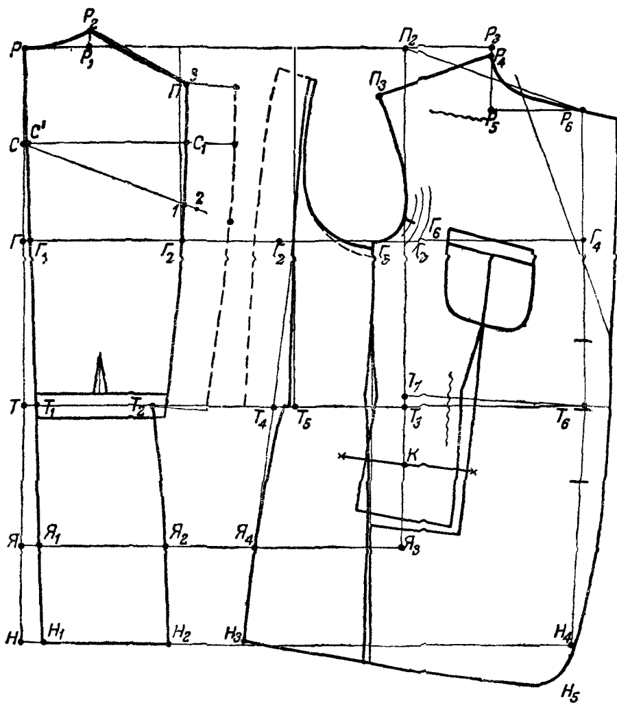
Рис 29 Чертеж пиджака
