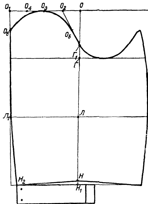
Рис. 74а. Чертеж рукава конькобежного костюма
