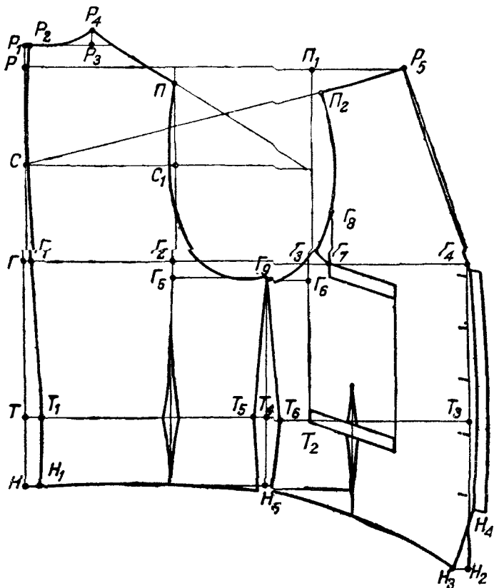
Рис. 79. Чертеж жилета
