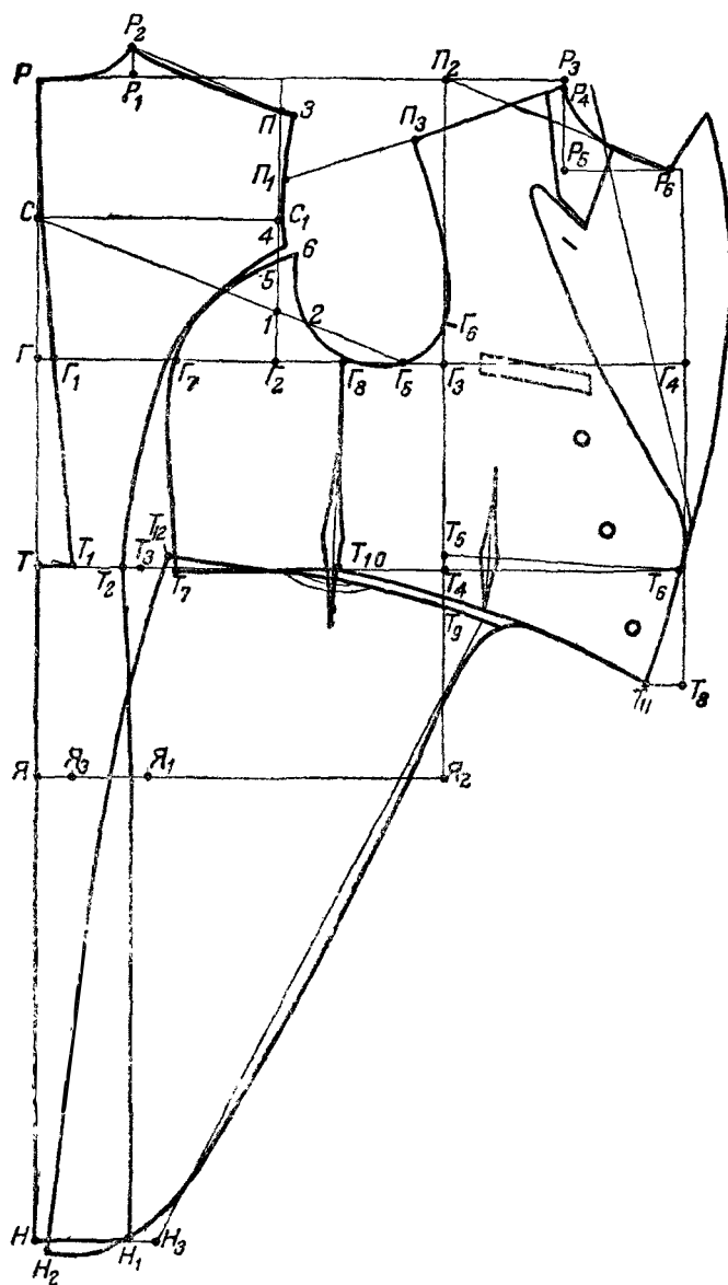
Рис. 103. Чертеж фрака
