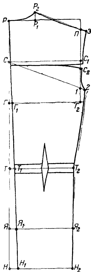
Рис. 26. Чертеж спинки пиджака фантази
