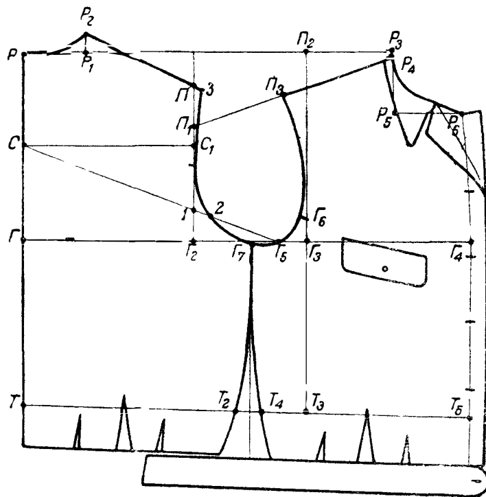
Рис. 76. Чертеж блузы лыжного костюма
