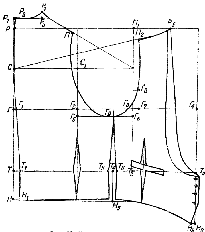
Рис. 83. Чертеж фрочного жилета
