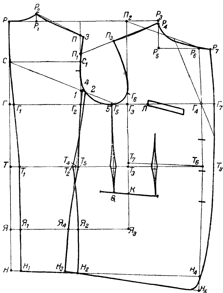
Рис. 14. Чертеж полы и спинки однобортного пиджака
