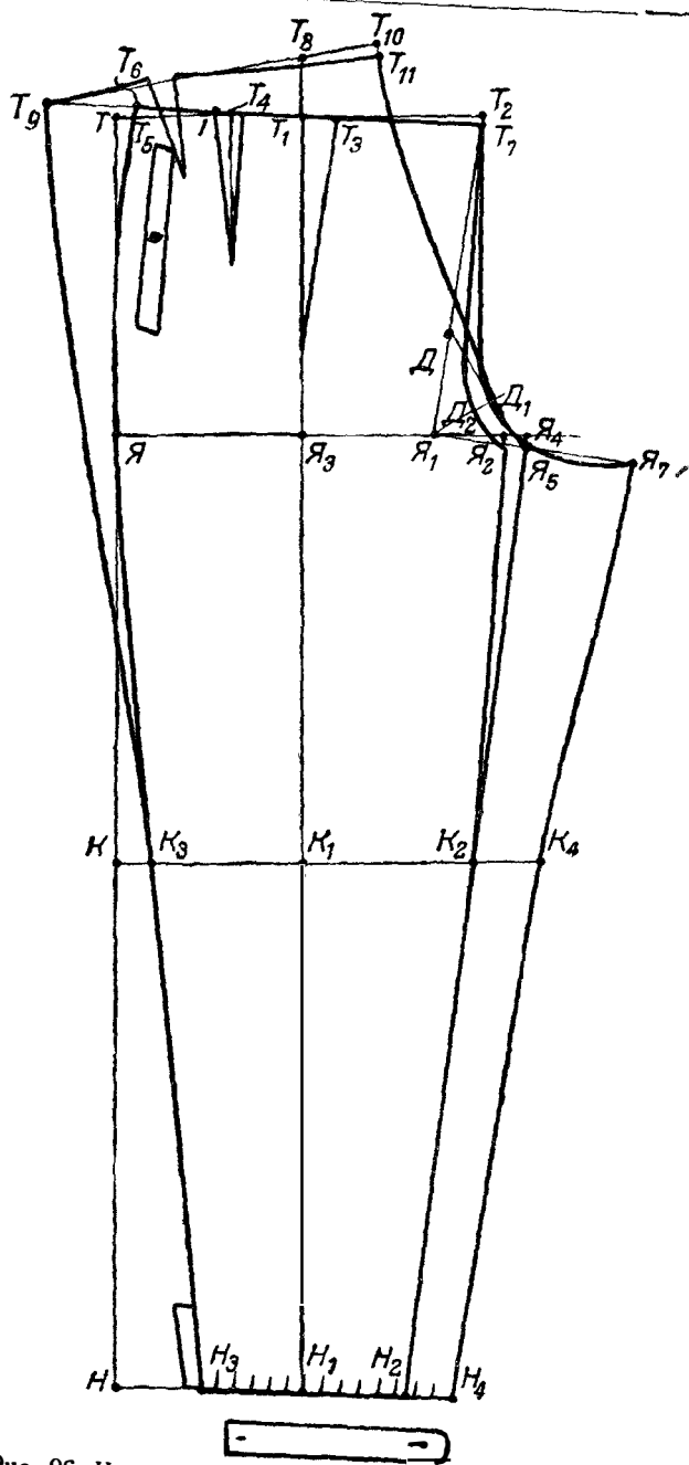
Рис. 96. Чертеж брюк для конькобежного спорта
