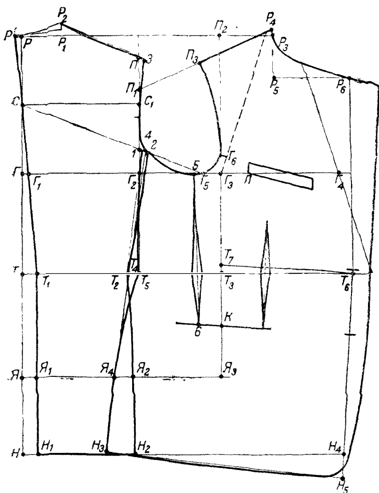
Рис. 33. Чертеж пиджака на перегибистую фигуру
