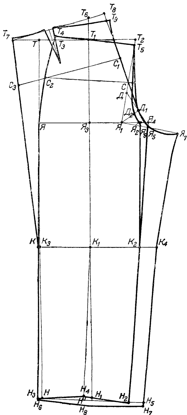
Рис. 90. Чертеж брюк на фигуру с X-образными ногами
