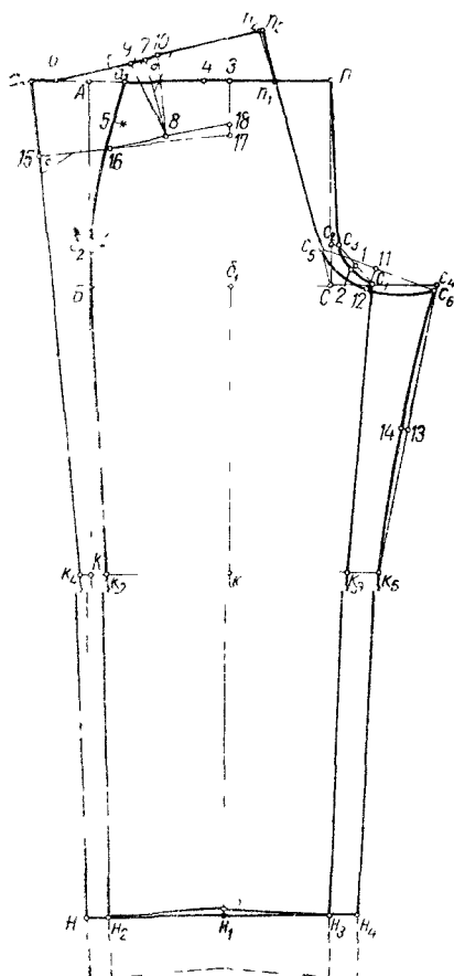
Рис. 5 Чертеж брюк обычного типа. Передняя и задняя половинки
