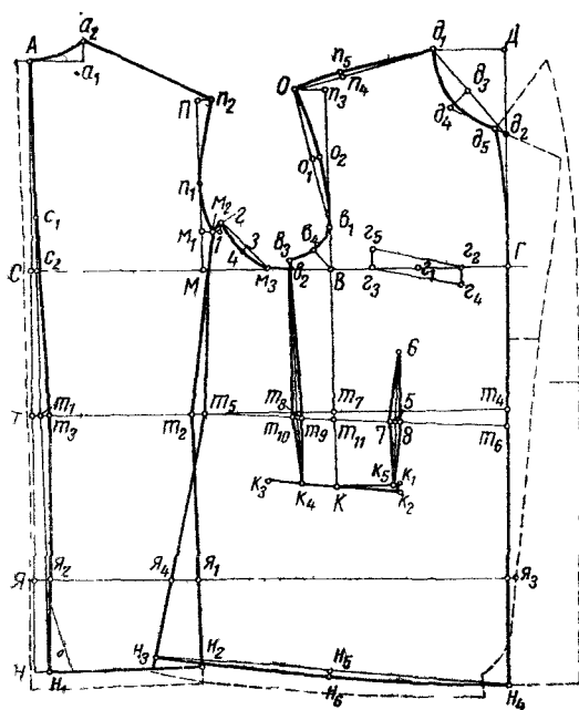
Рис. 1 Чертеж спинки и полы пиджака
