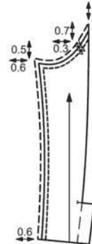
Рис. 11 Переднее полотнище юбки
