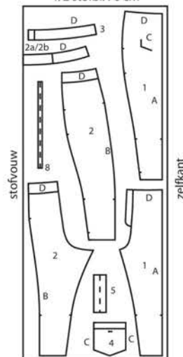
ОСНОВНОЙ МАТЕРИАЛ, РАЗМЕРЫ 40–54
