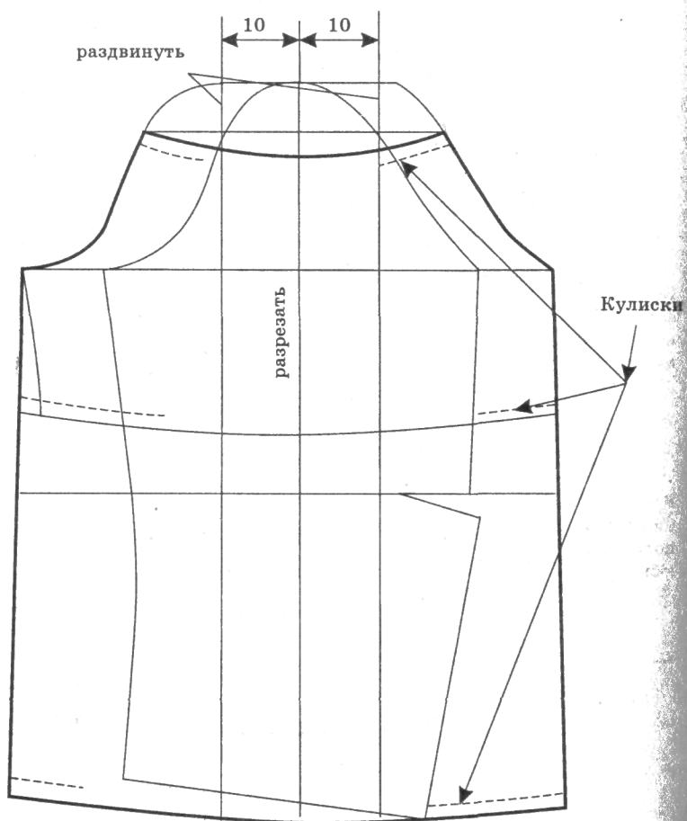
Рукав (по 2 детали)
