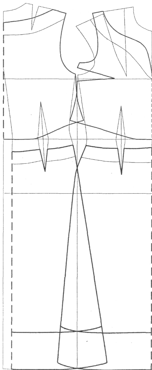
Чертеж выкройки блузы и юбки
