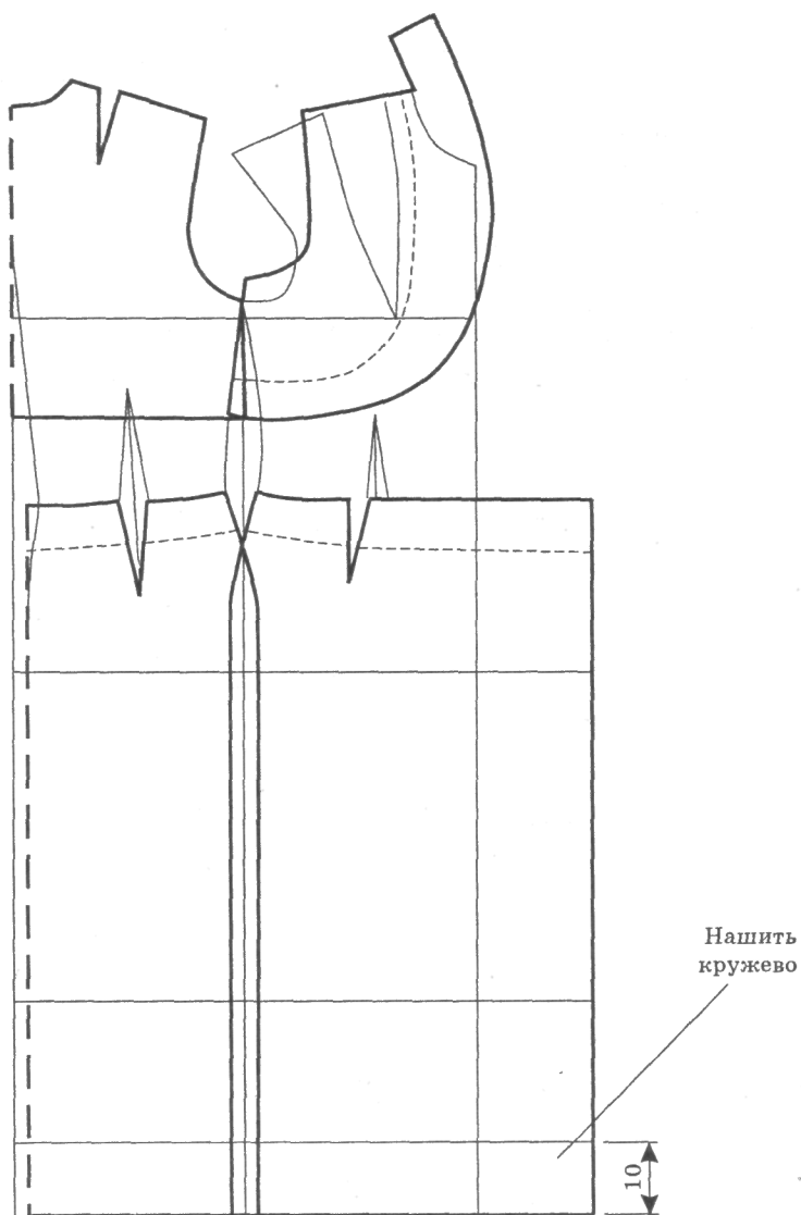
Болеро и юбка с запахом
