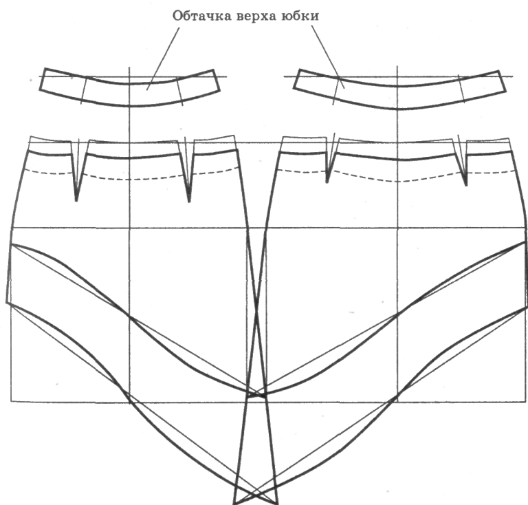
Заднее полотнище юбки
