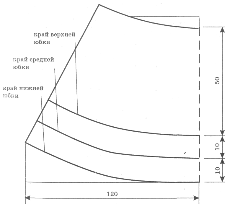
Переднее и заднее полотнища юбок
