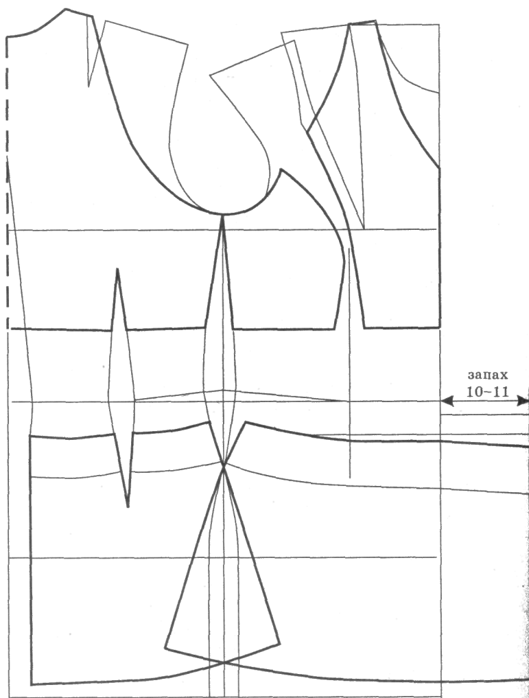
Топ и юбка с запахом
