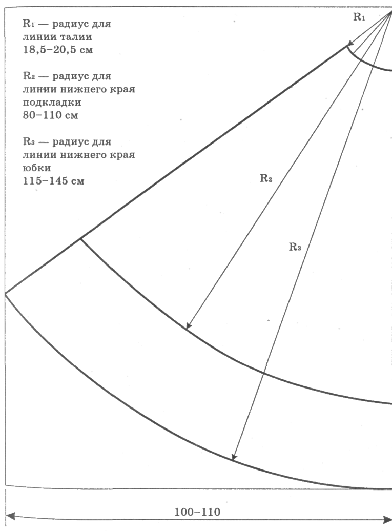
Переднее и заднее полотнища юбки
