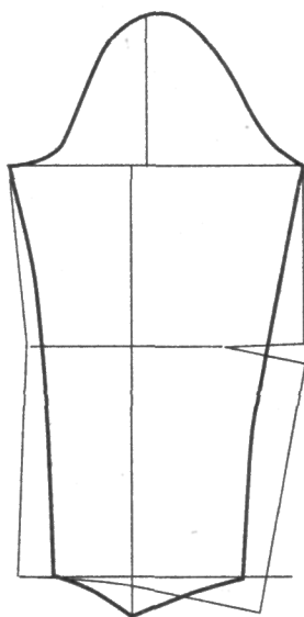
Рукав платья (левый)
