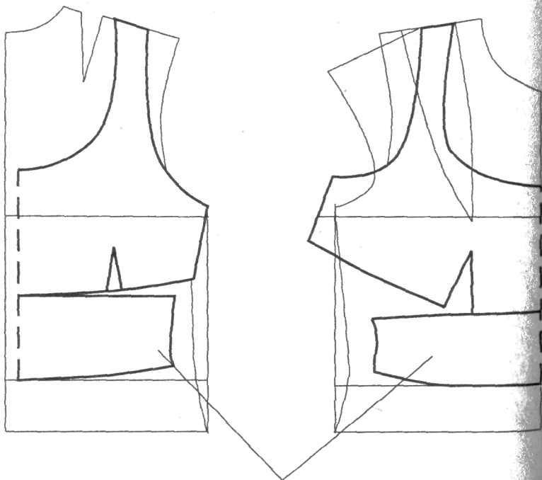
Детали из прозрачной эластичной ткани
