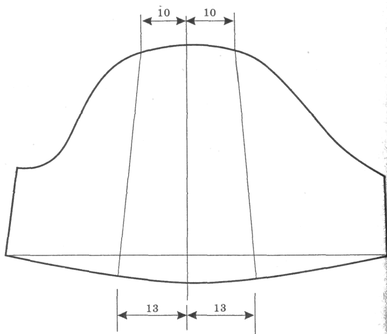
Верхняя деталь рукава
