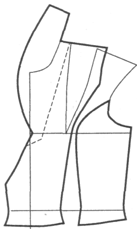
Средняя и боковая деталь левой полочки
