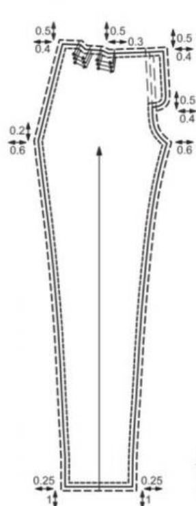
Рис. 9 Бочок, цельнокроеный с подкладкой кармана
