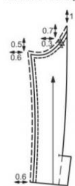
Рис. 11 Переднее полотнище юбки
