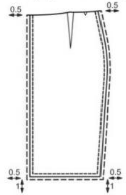
Рис. 11 Переднее полотнище юбки
