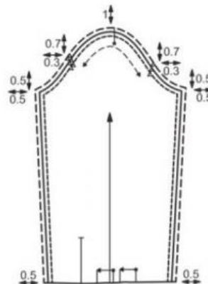
Рис. 4 Одношовный рукав
