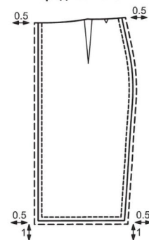
Рис. 11 Переднее полотнище юбки
