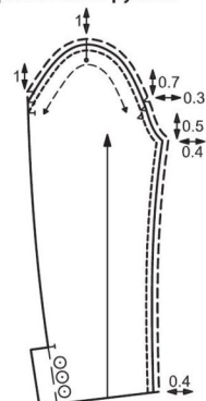
Рис. 10 Заднее полотнище юбки
