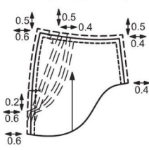
Рис. 9 Бочок, цельнокроеный с подкладкой кармана
