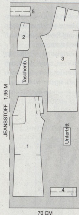
ZUSCHNEIDEPLAN
