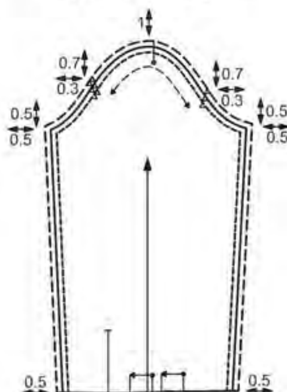
Рис. 4 Одношовный рукав
