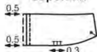
Рис. 2 Воротник
