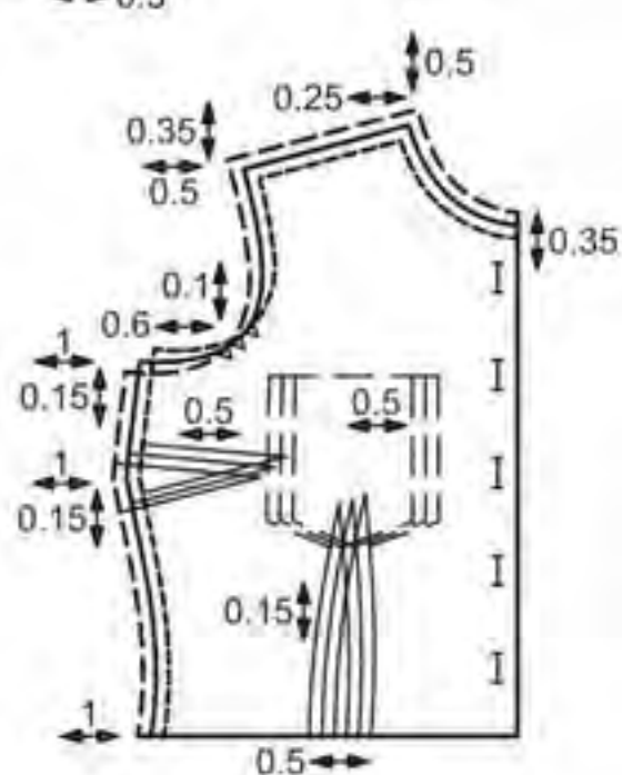
Рис. 3 Перед
