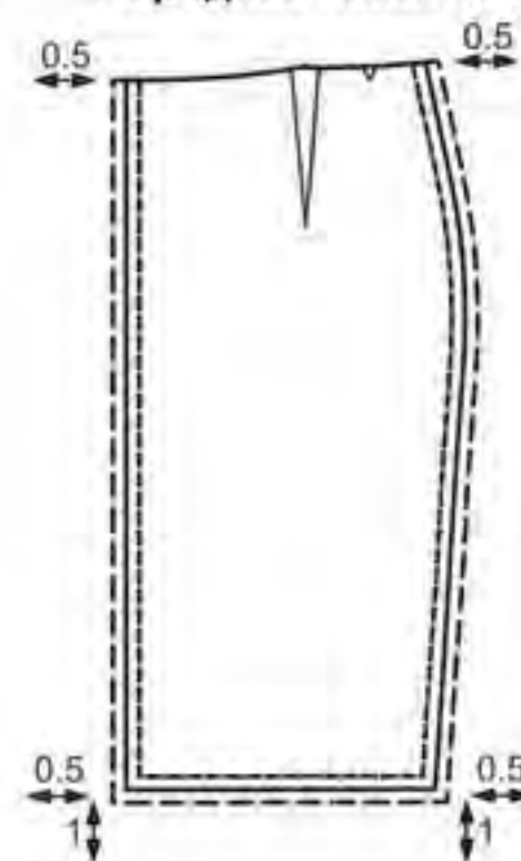
Рис. 11 Переднее полотнище юбки
