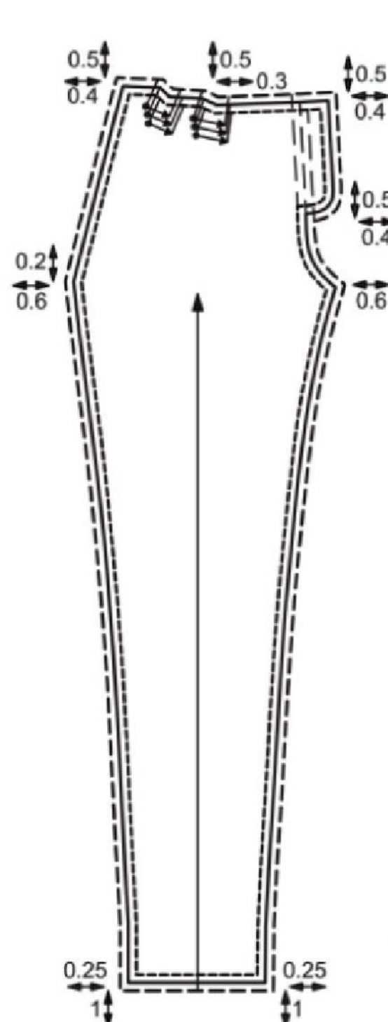
Рис. 8 Передняя половинка брюк
