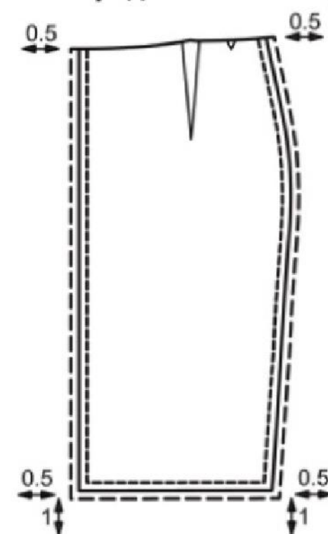
Рис. 11 Переднее полотнище юбки
