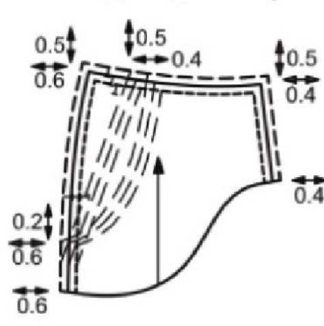
Рис. 9 Бочок, цельнокроеный с подкладкой кармана
