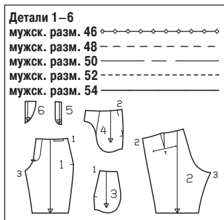
План раскладки при ширине ткани 145 см
