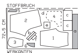
План раскладки при ширине ткани 145 см
