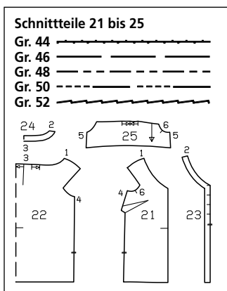
Schnittübersicht
