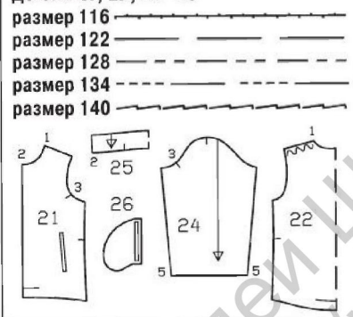
Выкройка с красными контурами на листе выкроек С Детали 21, 22, 24–26
